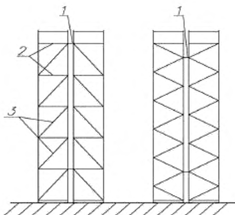
Рисунок 14 – Схема установки межрамных связей
