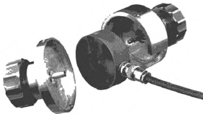
Рисунок В.9 — Токосъемник между двумя половинами коаксиального адаптера
