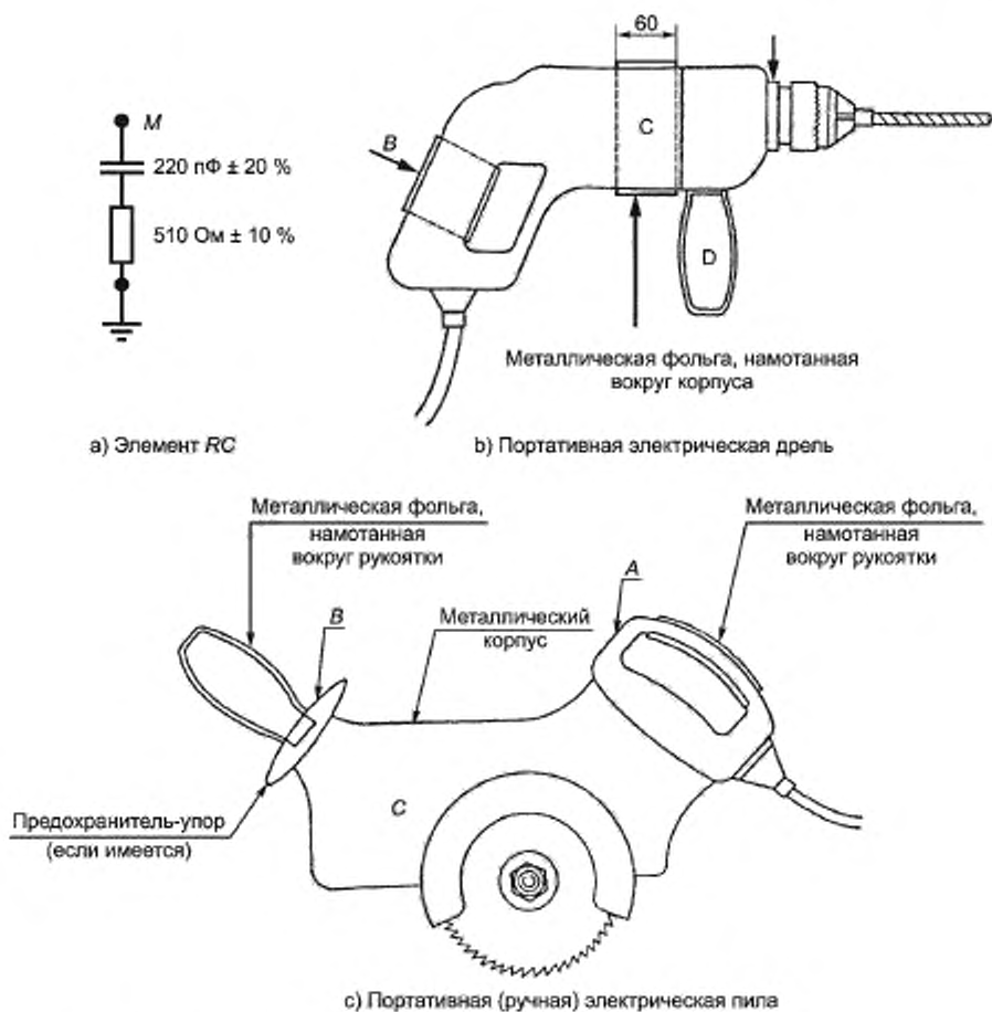
Рисунок 10 — Применение эквивалента руки
