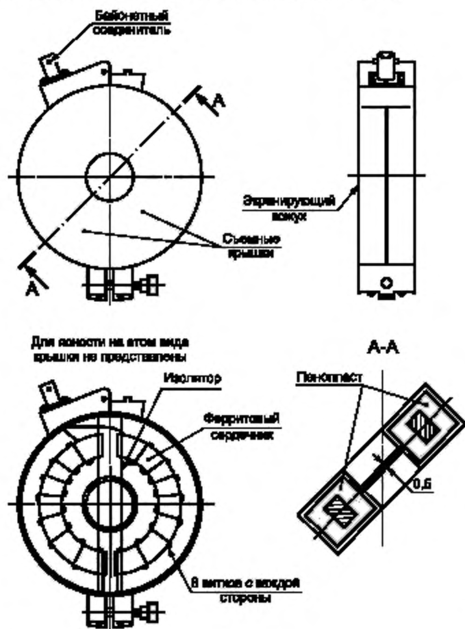
Рисунок В.1 — Типовая конфигурация пробника тока
