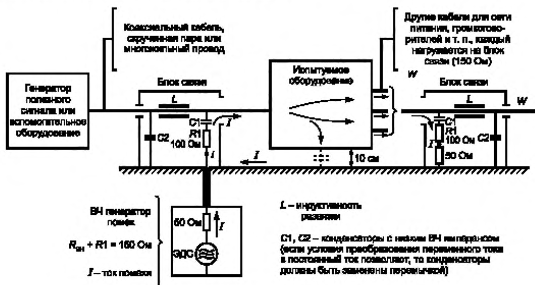
Рисунок D.1 — Принцип испытаний на помехоустойчивость при инжекции тока помех
