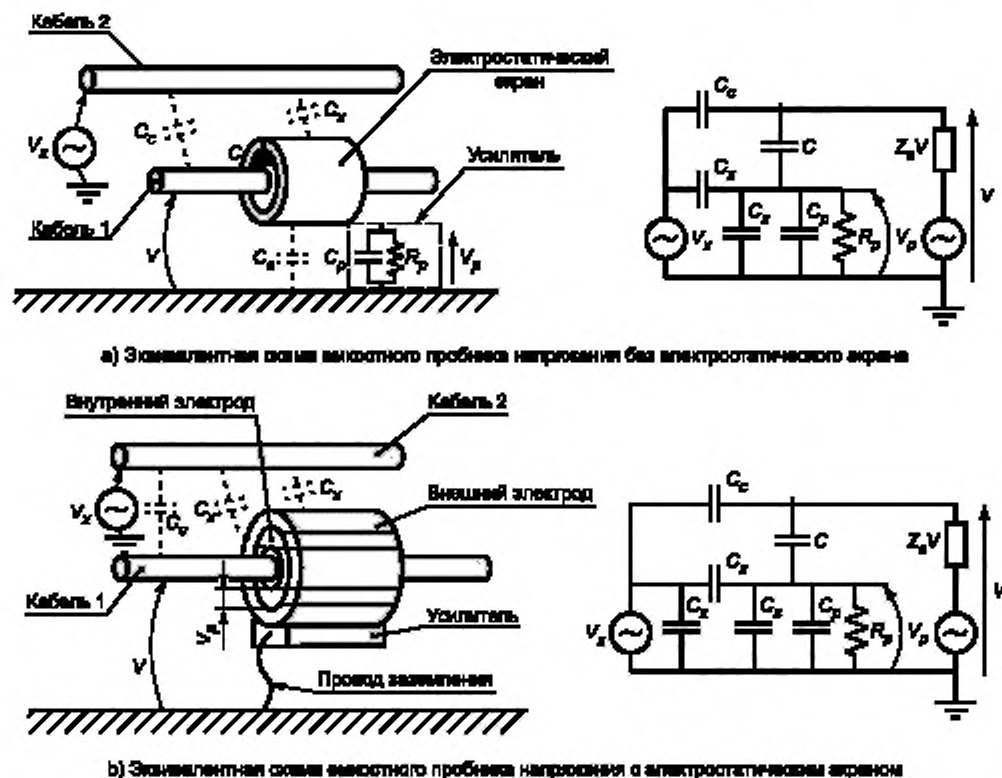
Рисунок G.4 — Модель электростатической связи и эквивалентная схема для емкостного пробоя напряжения
