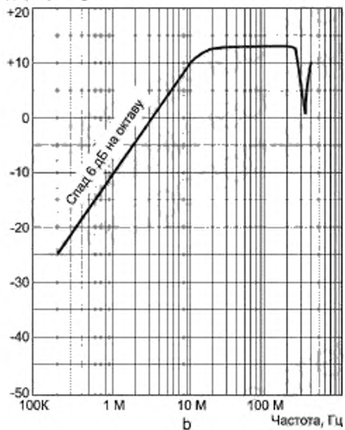
Рисунок В.3 — Зависимость передаточного полного сопротивления типовых пробников тока от частоты
