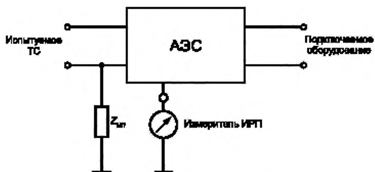
а) Схема подключения АЭС
