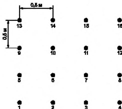
Рисунок D.1 — Положения измерительной антенны (датчика) в плоскости однородного поля
