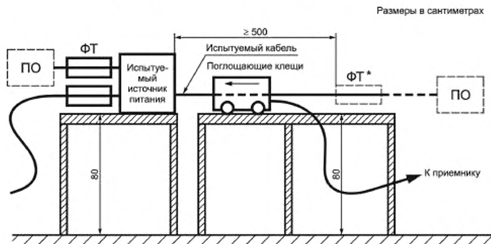
Рисунок 2 — Испытательная установка для измерения мощности промышленных радиопомех
