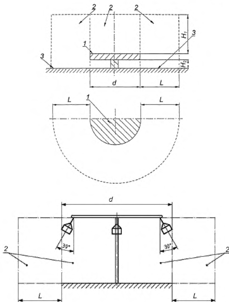
1 — платформа, 2 — зона безопасности; 3 — зона приземления. d — диаметр платформы; H_1 — высота зоны безопасности; H_2 — расстояние от нижней плоскости платформы до поверхности игровой площадки; L — ширина зоны безопасности и зоны приземления
