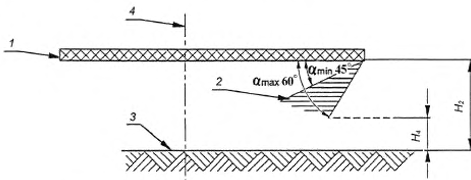
1- платформа карусели; 2 — зона допустимого перемещения защитной юбки карусели; 3 — поверхность игровой площадки; 4 — ось вала; H_2 — расстояние от нижней плоскости платформы до поверхности игровой площадки, 110 \leq H_2 \leq 400 мм, а — угол отклонения защитной юбки при вращении карусели; H_4 — расстояние от нижнего края защитной юбки до поверхности игровой площадки, 60 \leq H_4 \leq 110 мм
