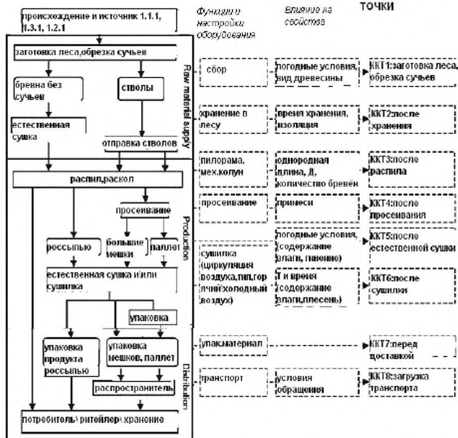
Схема 3 – Пример описания процесса производства и цепочки поставки с факторами, влияющими на качество, и критическими контрольными точками
