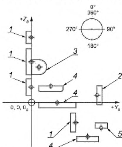
1 — задняя опора (ЗО); 2 — передняя опора (ПО); 3 — боковая опора (БО); 4 — нижняя опора (НО); 5 — верхняя опора (ВО)
