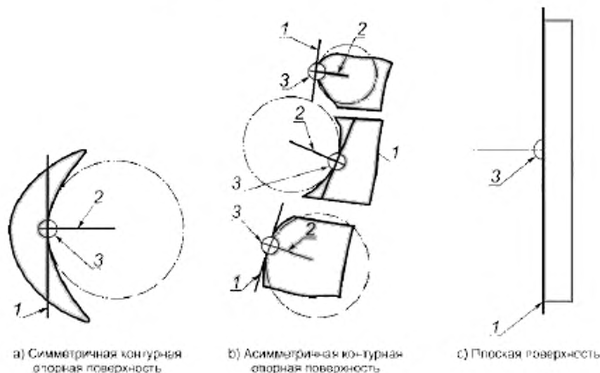
Рисунок 4 — Пример базовых плоскостей опорной поверхности для контурных и плоской поверхностей
