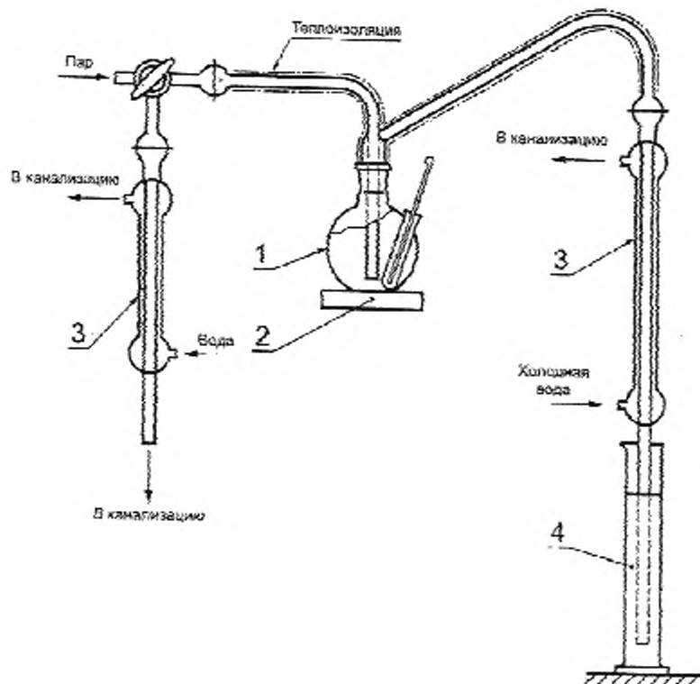
1 – дистилляционная колба; 2 – электроплитка; 3 – холодильник; 4 – приемный цилиндр
