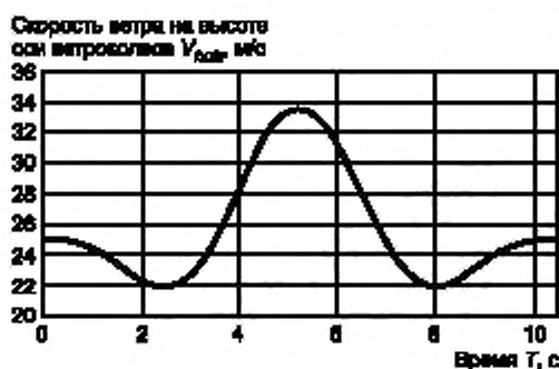
Рисунок 2 — Пример экстремального рабочего порыва
