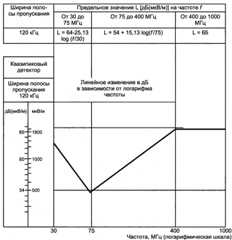
Рисунок А.5 — Контрольные предельные уровни широкополосных электромагнитных полей, создаваемых электрическими/электронными сборочными узлами
