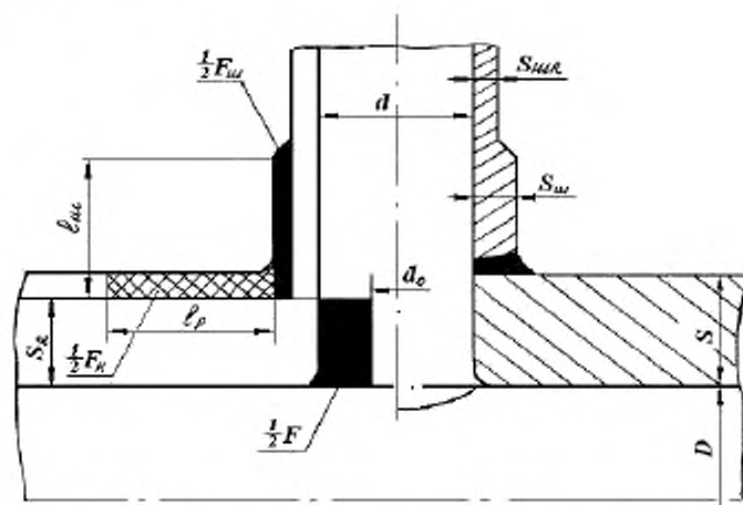
Рисунок 5.1 – Схема компенсации площадей при укреплении отверстия
