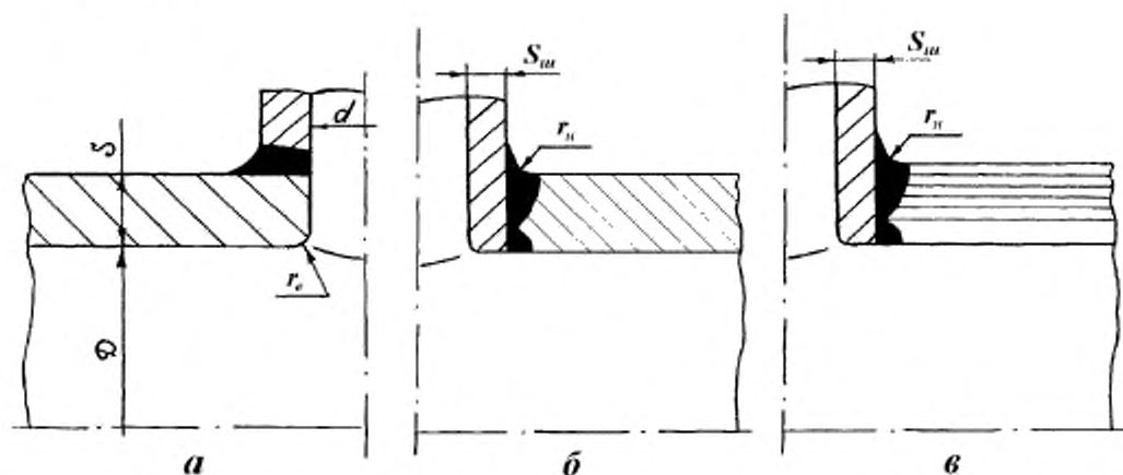
a – штуцер, приваренный к наружной поверхности обечайки (только для кованого корпуса); b – штуцер, вваренный в стенку обечайки; v – штуцер, вваренный по всей толщине многослойной обечайки
