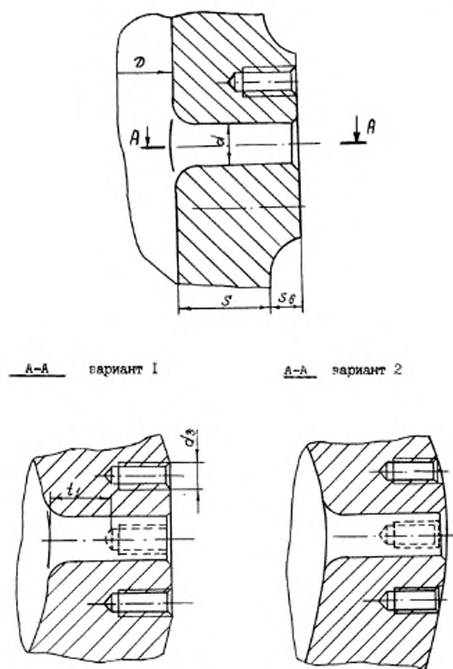
Рисунок 4.4 – Размещение резьбовых гнезд для крепежных элементов
