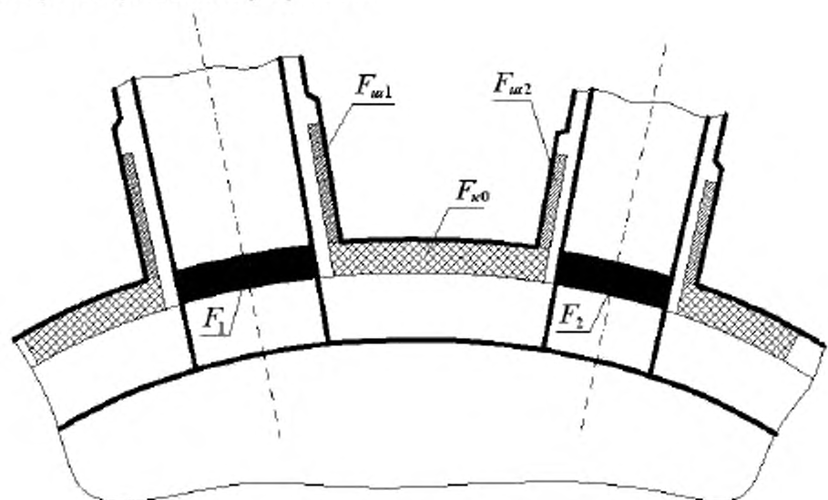
Рисунок 5.2 – Схема укрепления взаимовлияющих отверстий
