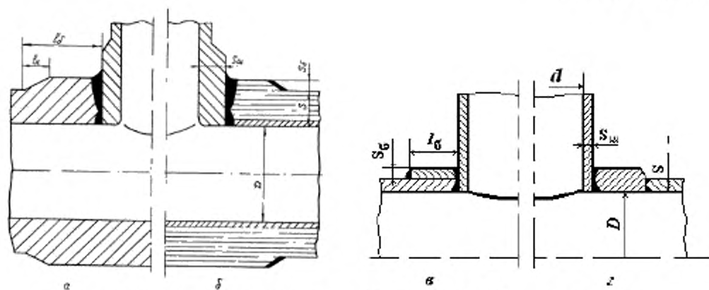
Рисунок 4.1 – Способы укрепления отверстий в обечайке (днище)
