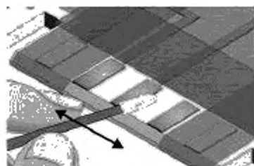
Рисунок 36 с – Удаление припоя
