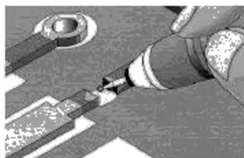
Рисунок 26 б – Пропил для размыкания печатного проводника
