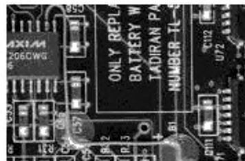
Рисунок 45 д – Приклеивание провода кусочками липкой ленты
