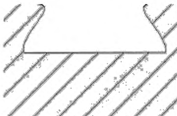
Рисунок 9 б – Подрез для увеличения механической прочности
