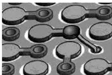
Рисунок 44 в – Припаивание перемычки из фольги к металлизированному отверстию, соединенному площадкой BGA
