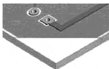
Рисунок 11 с – Фрезерование уступа в кромке имплантанта
