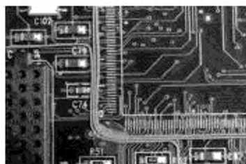
Рисунок 45 а – Прокладка перемычки на поверхности платы
