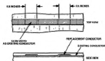
Рисунок 24 ф – Технические данные по замене
