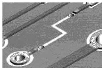
Рисунок 22 b – Сверление сквозных отверстий рядом с проводником
