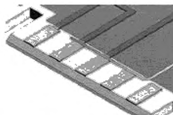
Рисунок 36 д – Припаивание провода по кромке металлируемых концевых контактов
