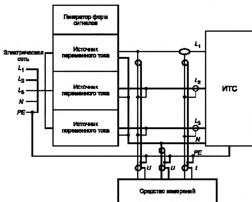
Рисунок 1 — Схема испытательной установки с использованием однофазного ИГ
