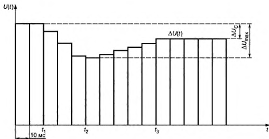
Рисунок 2 — Схема определения огибающей среднеквадратичных значений напряжения
