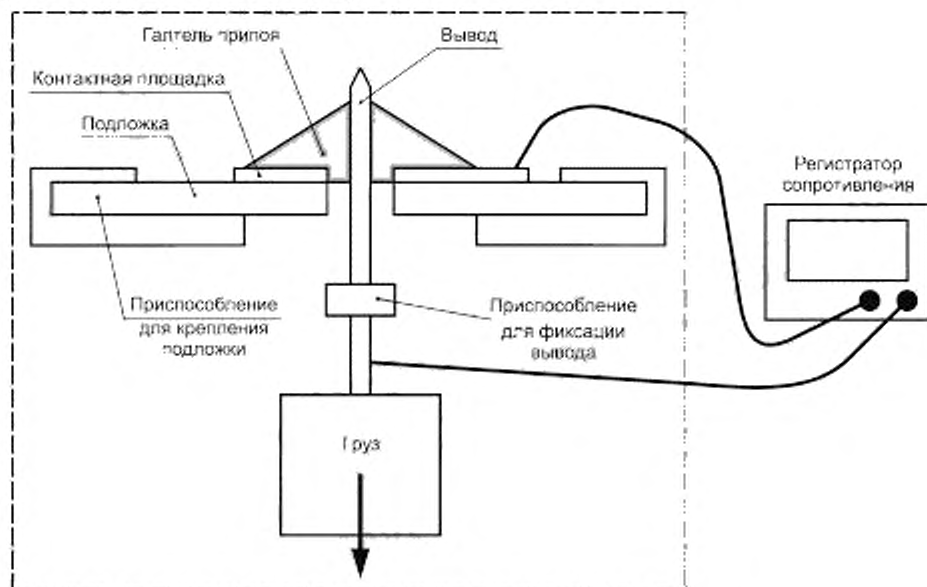
Рисунок G.1 — Испытание на сопротивление ползучести
