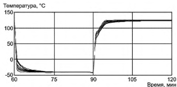
а) Распределение температуры (0 подложек)
