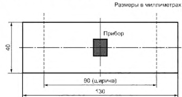
Рисунок 3 — Пример монтажа поверхностно монтируемого прибора для проведения испытаний на устойчивость при монотонном и циклическом изгибах
