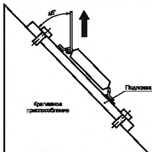
Рисунок 8 — Испытание прочности на отрыв
