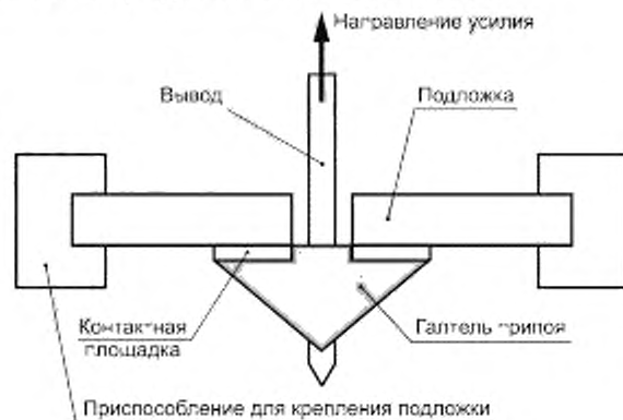
Рисунок F.1 — Испытание прочности на отрыв
