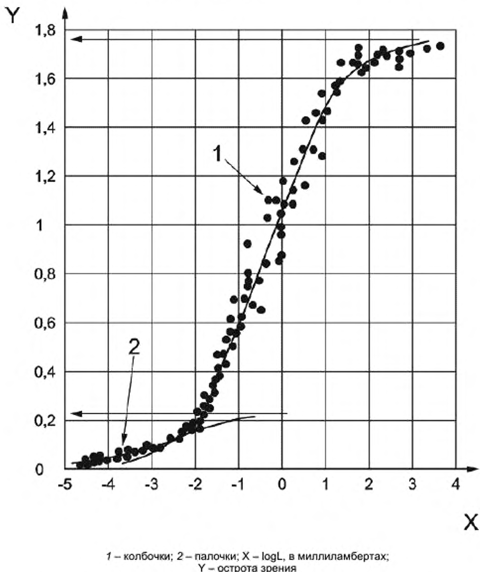
Рисунок 5 – Для задач распознавания на остроту зрения влияет уровень фоновой яркости
