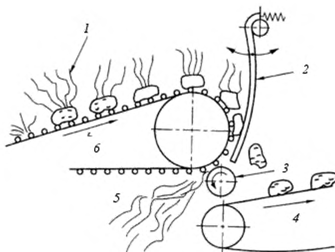
1 – ботва, 2 – пальцы для отделения ботвы, 3 – ролик для отделения ботвы, 4 – цепь конвейера, 5 – выброс ботвы, 6 – подъемная цепь Рисунок В.3а – Отделение ботвы при помощи ролика
