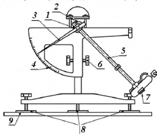
Рисунок 2 – Устройство для измерения трения
