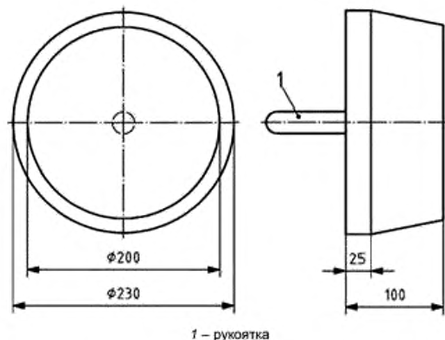
Рисунок Г.5 – Щуп В (большой) для определения застывания головы или шеи пользователя в отверстиях
