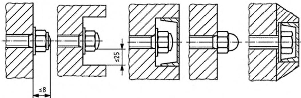
Рисунок 2 – Защита болтовых соединений
