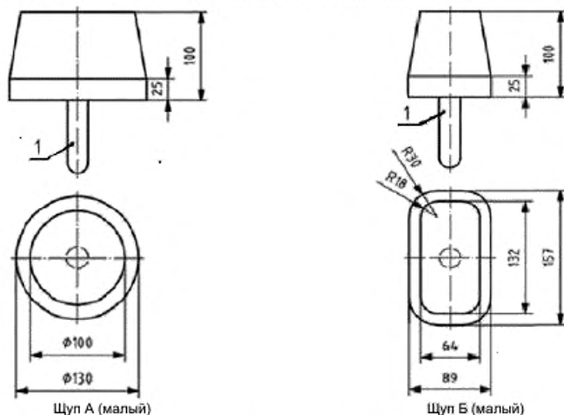
Рисунок Г.4 – Щупы (малые) для определения застывания головы или шеи пользователя в отверстиях
