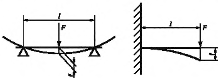
Рисунок 9 — Пример нагружения элементов тренажера
