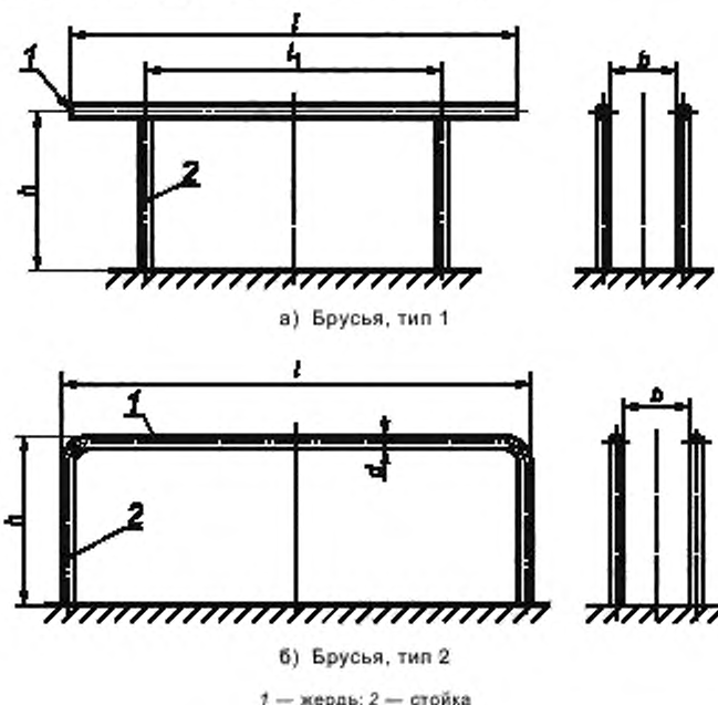
Рисунок 3 — Параллельные брусья
