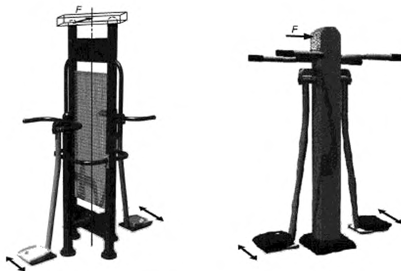
Рисунок Е.1 — Примеры приложения нагрузки
