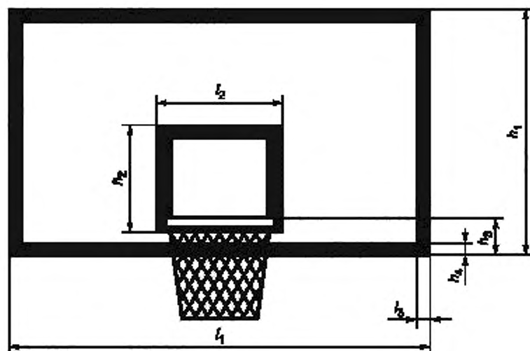
Рисунок 10 — Рекомендуемые размеры баскетбольного щита и размеры маркировки
