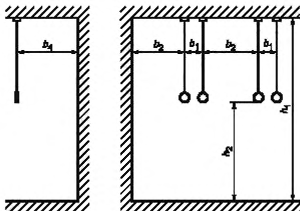
Рисунок 6 — Установочные размеры для колец
