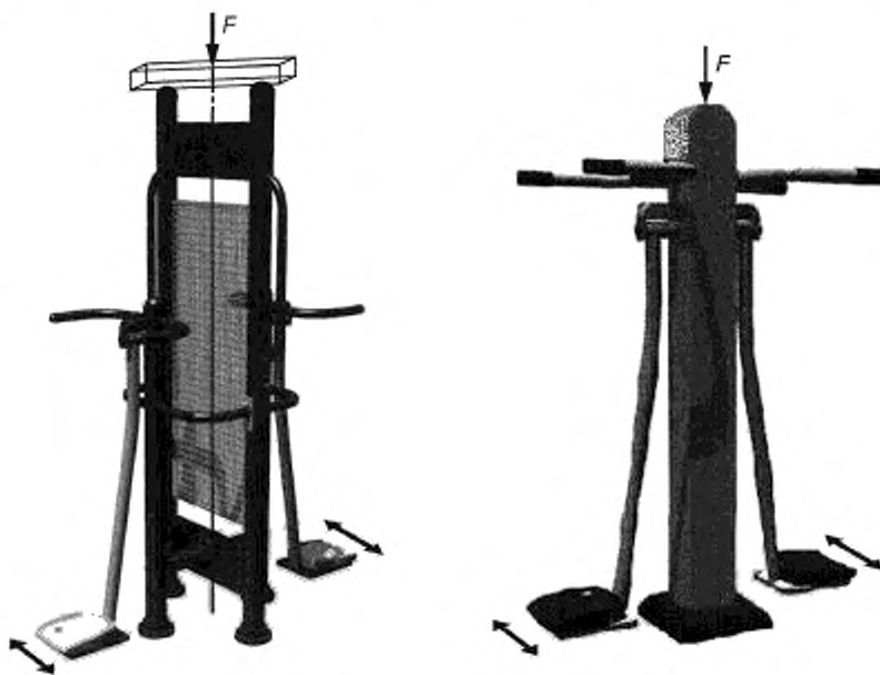
Рисунок Е.2 — Примеры приложения нагрузки
