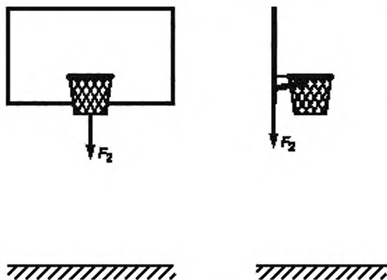
Рисунок Ж.4 — Нагружение при испытаниях на устойчивость
