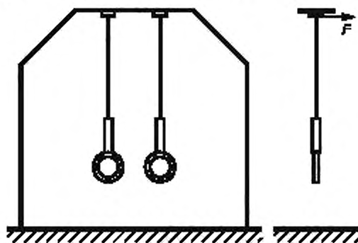
Рисунок В.2 — Схема приложения горизонтальной нагрузки
