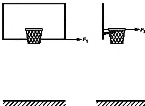
Рисунок Ж.3 — Нагружение при испытаниях на прочность
