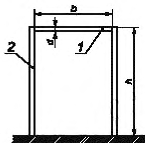
Рисунок 2 — Перекладина
