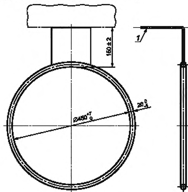
Рисунок 11 — Размеры баскетбольного кольца
