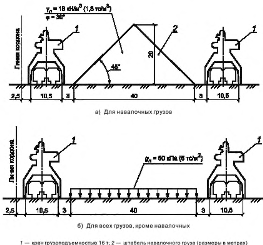
Рисунок 6.1 — Схемы нормативных нагрузок на прикормонной территории грузовых причалов
