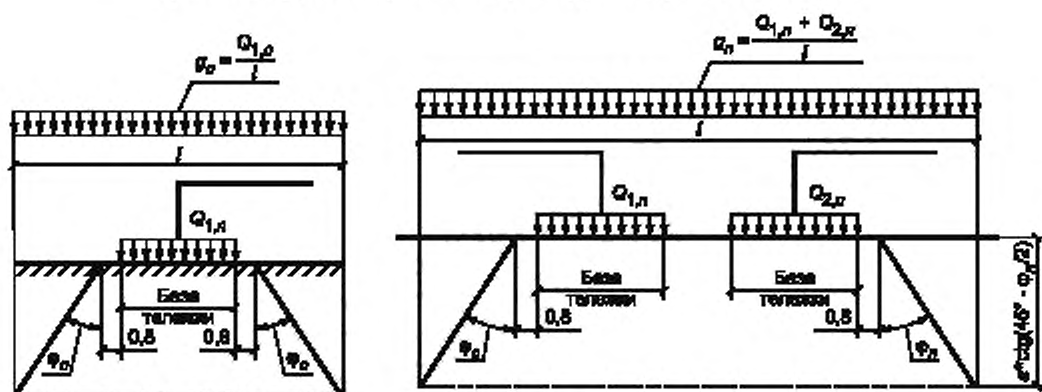
б) Схема распределения нагрузки вдоль грузового причала от ноги крана
