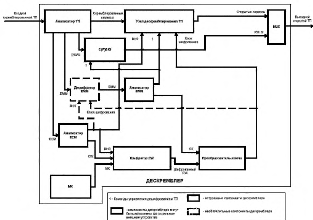
Рисунок 2 – Структурная схема МОД
