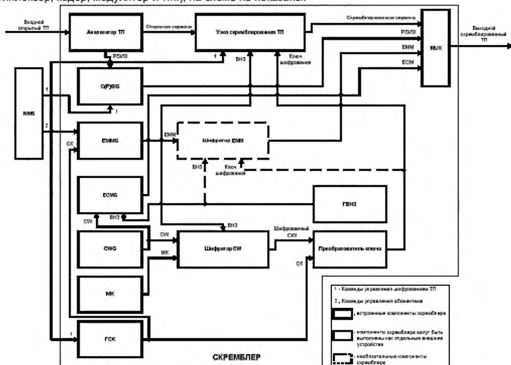
Рисунок 1 – Структурная схема передающей стороны СОД
