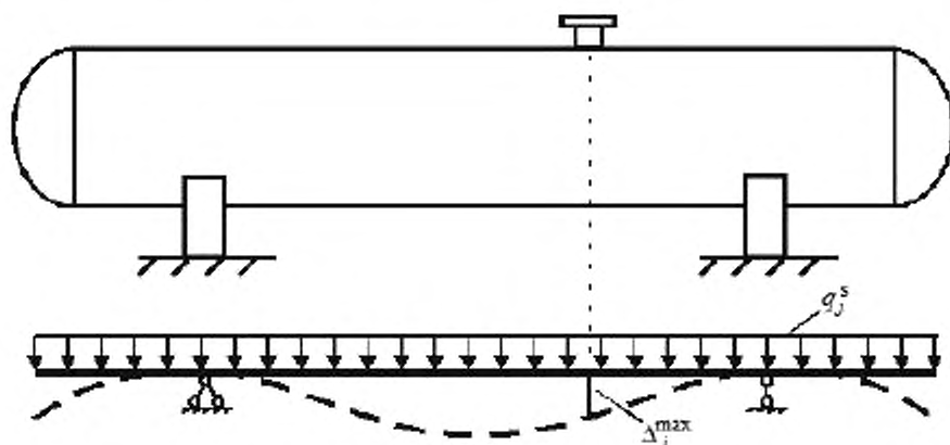
Рисунок 15 – Расчетная схема для определения перемещений штуцеров от сейсмического воздействия
