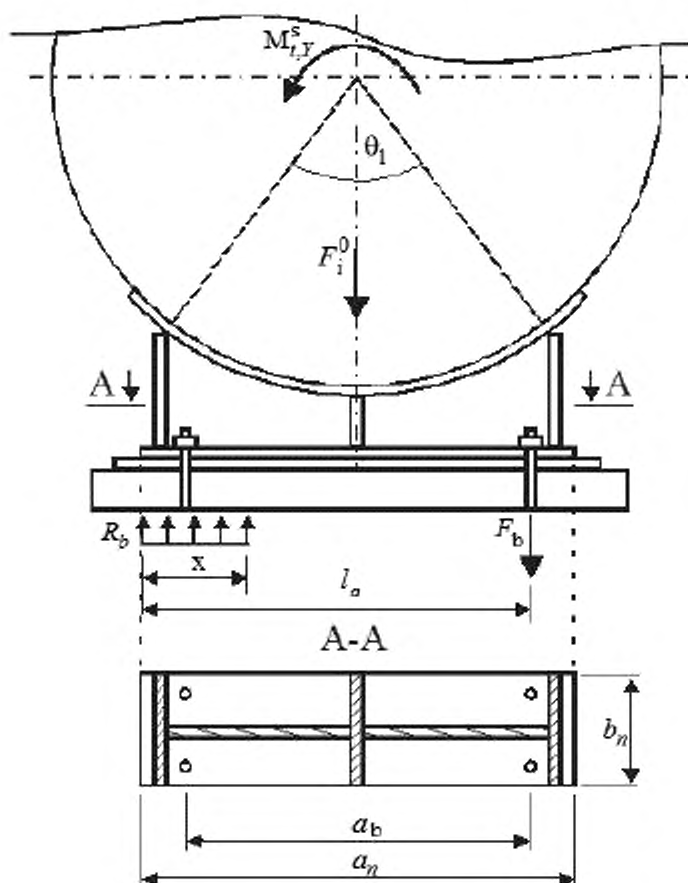
Рисунок 14 – Расчетная схема для определения нагрузки на анкерные болты
