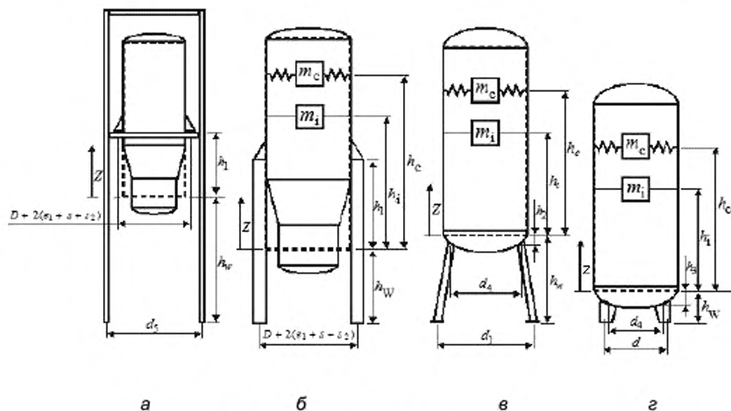
Рисунок 8 – Вертикальный сосуд
