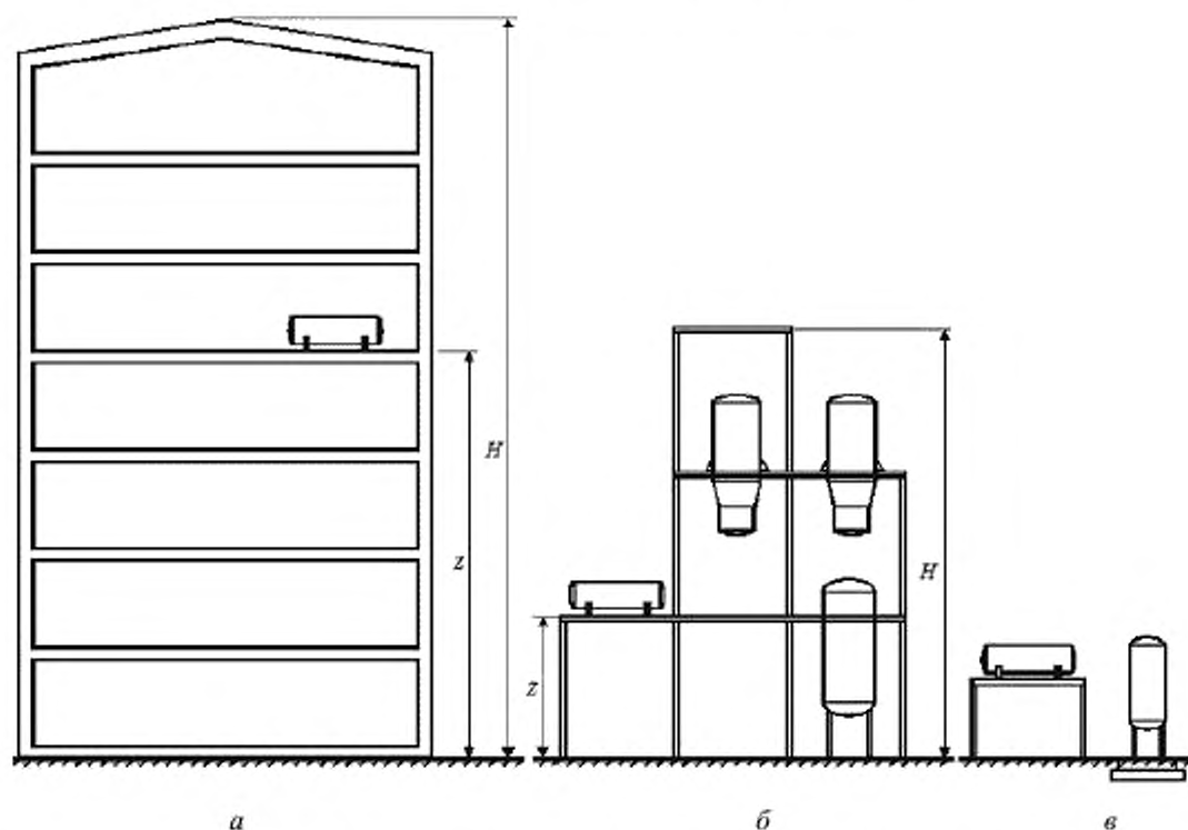
Рисунок 1 – Варианты установки сосуда
