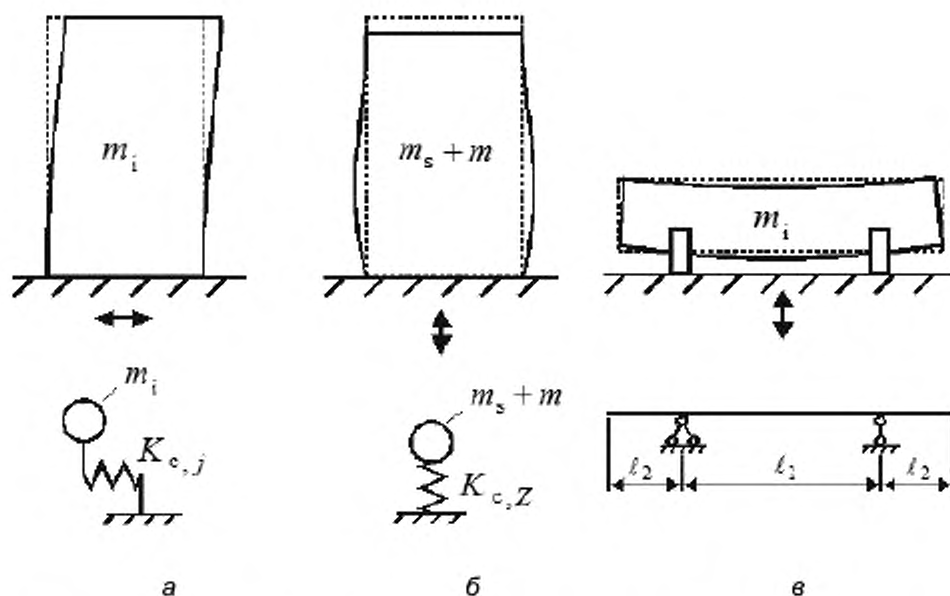
Рисунок А.1 – Формы колебаний сосудов и соответствующие расчетные модели
