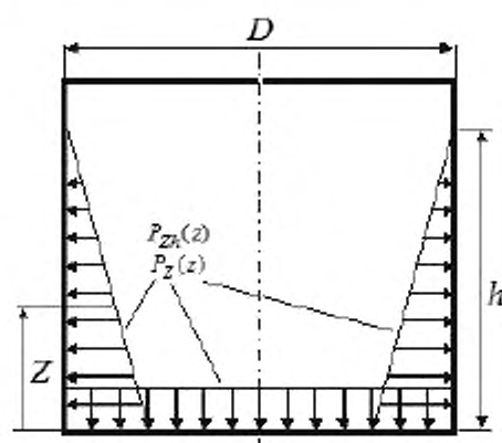
Рисунок 10 – Гидродинамическое давление на стенки и днище от сейсмического воздействия в вертикальном направлении
