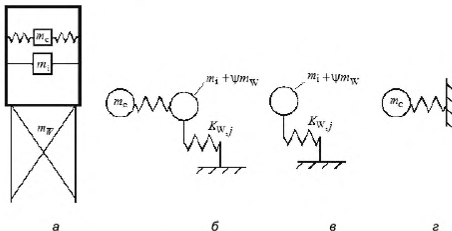
Рисунок 6 – Модель сосуда с учетом жесткости опорной конструкции при горизонтальном воздействии
