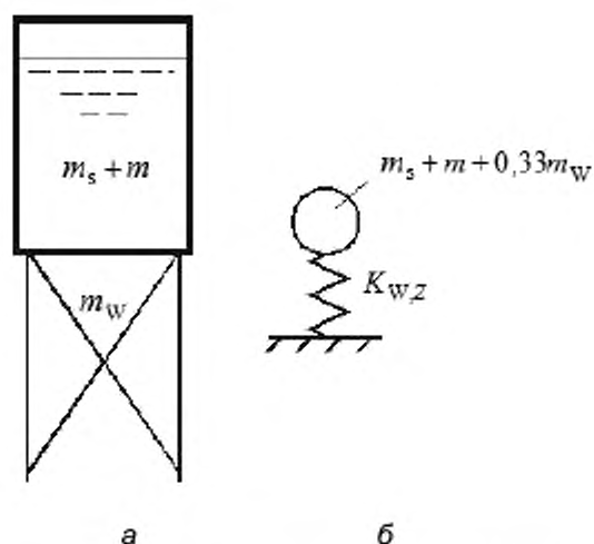
Рисунок 7 – Модель сосуда с учетом жесткости опорной конструкции при вертикальном воздействии
