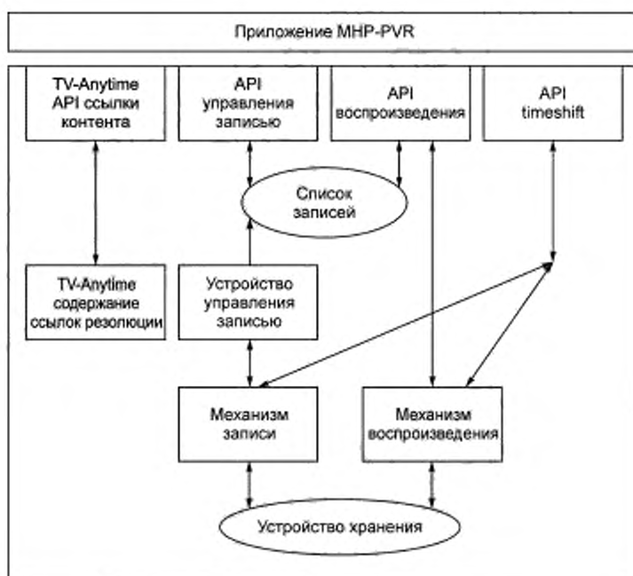
Рисунок 4 — Упрощенная архитектура MHP-PVR
