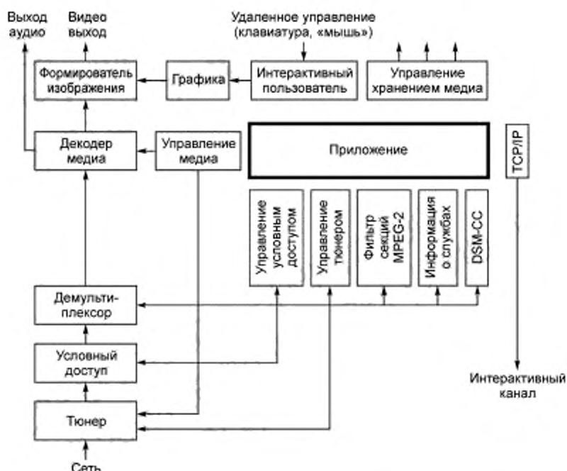
Рисунок 2 — Интерфейсы между приложениями MHP и системой MHP
