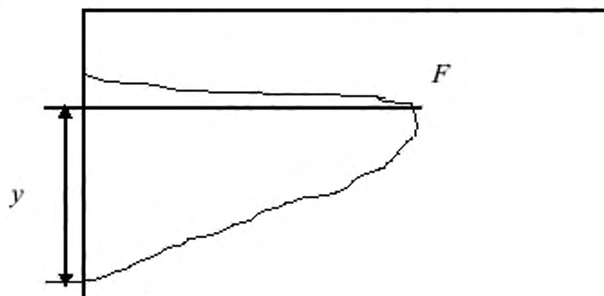
Рисунок 1 – Пример регистрационной кривой силы смещения
