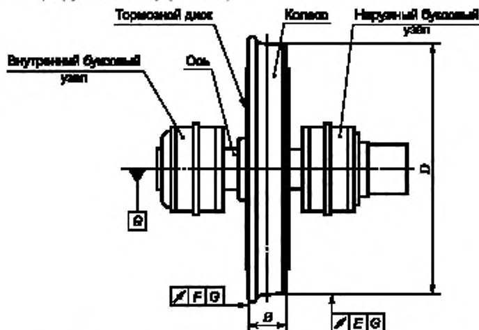
Рисунок 4 — Колесный узел колесного блока
