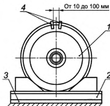
1 — колесная пара, 2 — основание; 3 — электроизоляционный материал; 4 — зажимы
