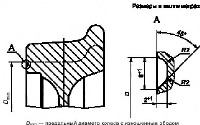
Рисунок 5 — Кольцевая проточка
