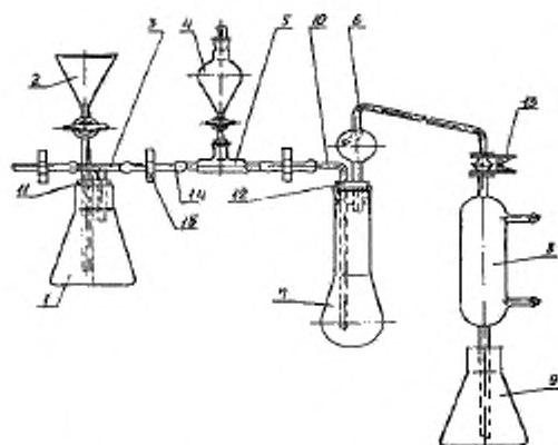
1 – коническая колба вместимостью 500 см 3 ; 2 – воронка с храником; 3 – Т-образная трубка; 4 – делительная воронка вместимостью 100 см 3 ; 5 – переходник; 6 – каллеуловитель; 7 – колба Кьельдаля вместимостью 250 см 3 ; 8 – шариковый холодильник; 9 – приемная мерная колба вместимостью 50 см 3 ; 10 – изогнутая трубка, 11, 12 – резиновые пробки; 13, 15 – зажим; 14 – резиновые трубки
