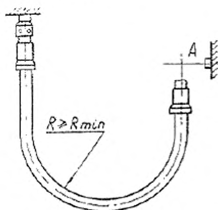
Рисунок А.2 – Резкий изгиб рукава у концевой арматуры
