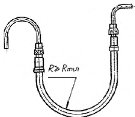
Рисунок А.4 – Двойной изгиб рукава
