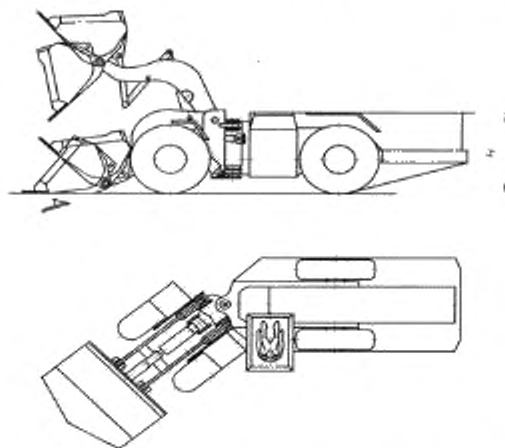
Рисунок 3 – Машина низкопрофильная с кабиной машиниста, вынесенной относительно продольной оси
