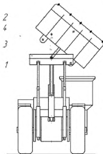
Рисунок 5 – Рабочее оборудование машины с ковшом для фронтальной и боковой разгрузки
