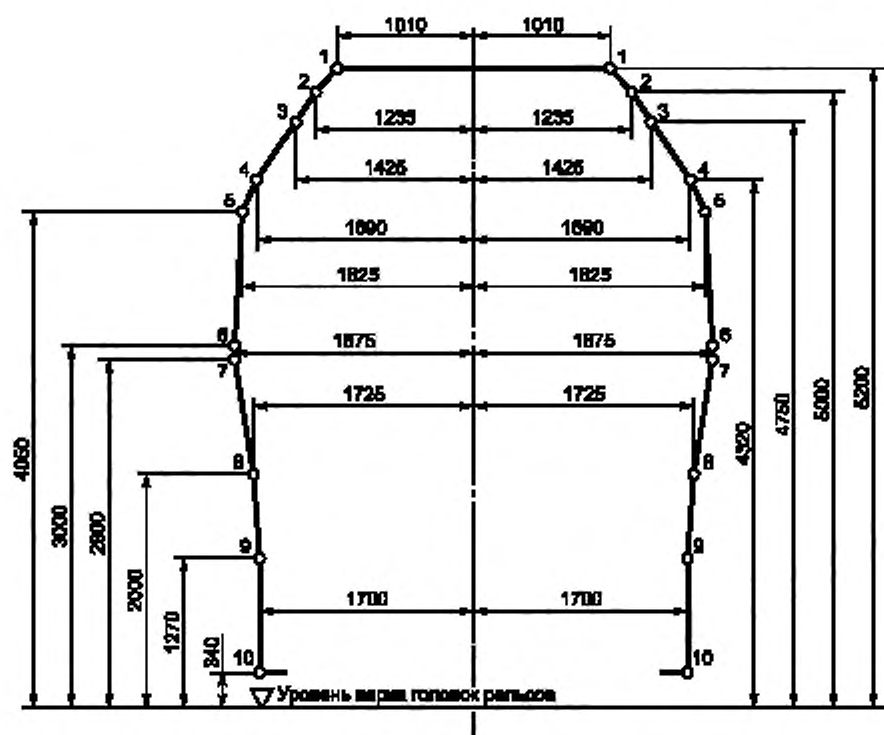
Рисунок 2 — Статический габарит T_{ц}
