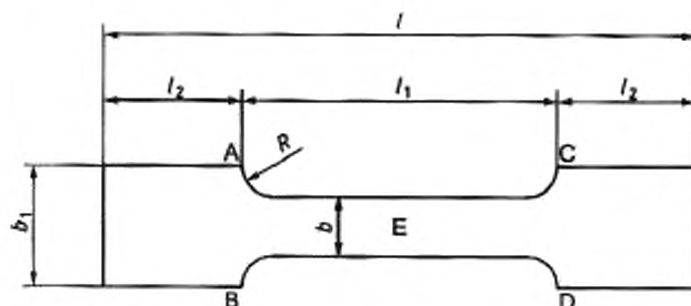
Рисунок 1— Форма испытуемого образца
