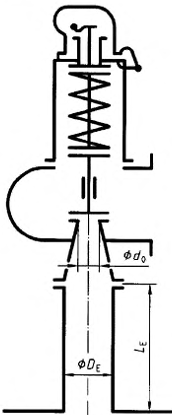
Рисунок 4.1 – Предохранительные клапаны
