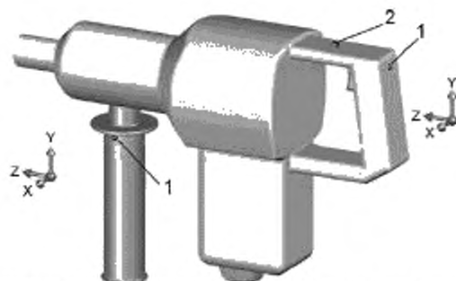
Рисунок 10 – Перфоратор
