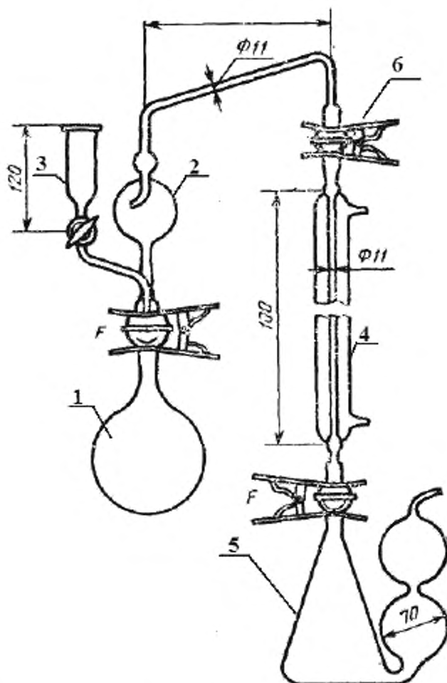
1 — колба для дистилляции; 2 — каплеотбойная головка; 3 — капельная цилиндрическая воронка; 4 — холодильник; 5 — коническая колба с боковыми шарообразными расширениями; 6 — пружинные зажимы
