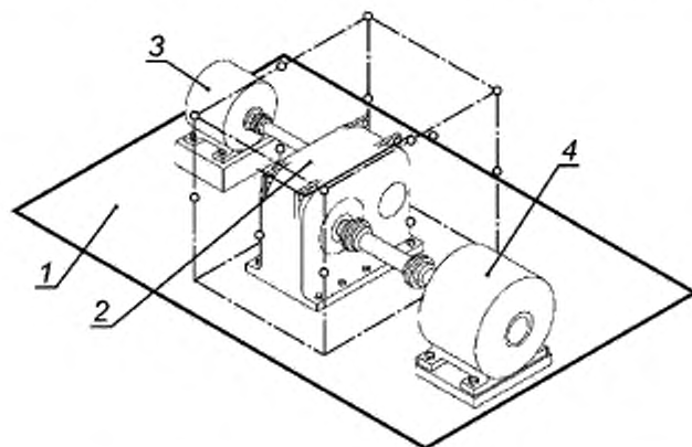
1 — пол; 2 — редуктор; 3 — двигатель; 4 — нагрузочное устройство ○ — точки измерений
