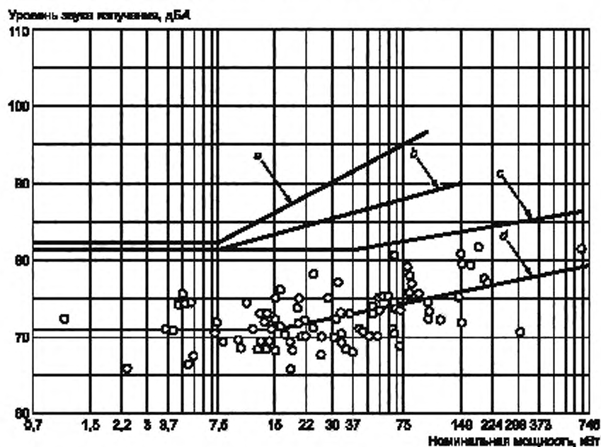
Рисунок В.2 — Типичные графики максимальных и средних уровней звука излучения мотор-редукторов, понижающих и повышающих одно-, двух- и трехступенчатых редукторов без вентилятора на холостом ходу или при малой нагрузке в зависимости от номинальной мощности
