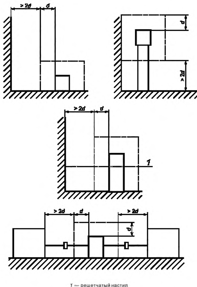
Рисунок 4 — Примеры установки редутора на полу и у стены
