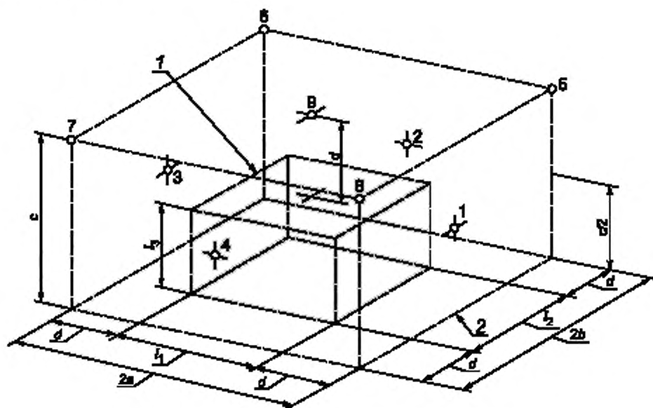
Рисунок 5 — Точки измерений для рисунка 4
