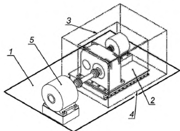
Рисунок 1 — Огибающий параллелепипед и измерительная поверхность для редуктора
