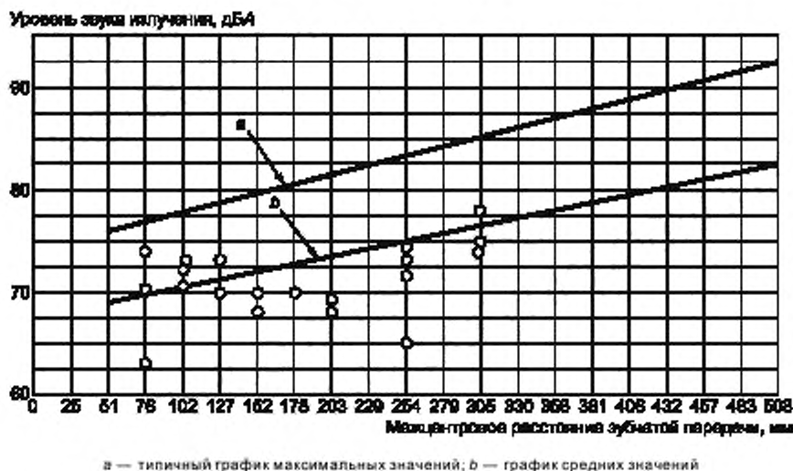
Рисунок В.7 — Уровень звука излучения одноступенчатого червячного редуктора с охлаждающим вентилятором при частоте вращения входного вала 1750 об/мин на расстоянии 1,5 м от корпуса на холостом ходу или при малой нагрузке, в зависимости от межцентрового расстояния
