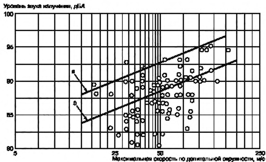
Рисунок В.3 — Уровень звука излучения быстроходных косозубых и двойных косозубых одноступенчатых редукторов на расстоянии 0,9 м от корпуса на холостом ходу или при малой нагрузке в зависимости от максимальной скорости по делительной окружности
