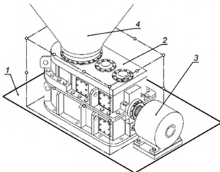
1 — пол; 2 — редуктор; 3 — двигатель; 4 — нагрузочное устройство ○ — точки измерений
