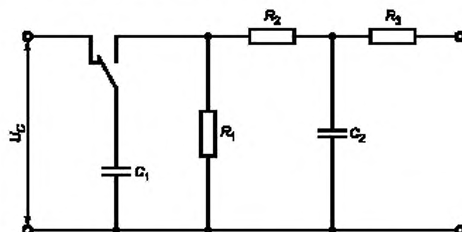
Рисунок К.1 — Схема испытательного импульсного генератора
