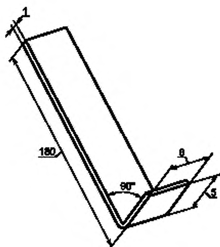
Рисунок 4 — Испытательный крюк
