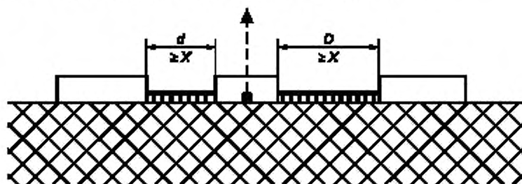
Рисунок E.8 — Промежуточная, несоединенная проводящая часть
