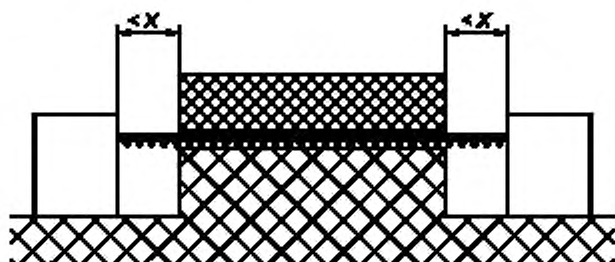
Рисунок E.5 — Несплошной стык с узкими канавками
