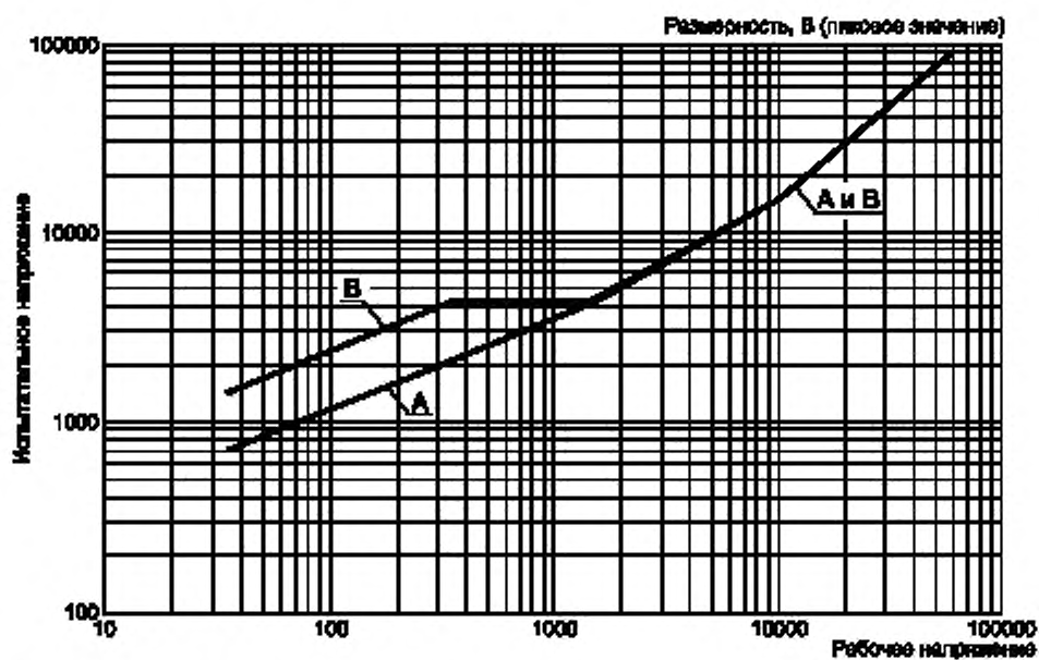
Рисунок 7 — Испытательное напряжение
