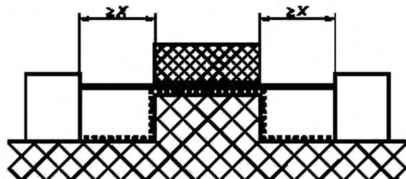
Рисунок E.6 — Несплошной стык с широкими канавками
