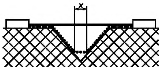
Рисунок E.3 — V-образная канавка
