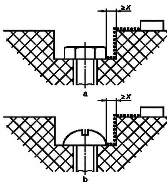
Рисунок Е.10 — Большое углубление
