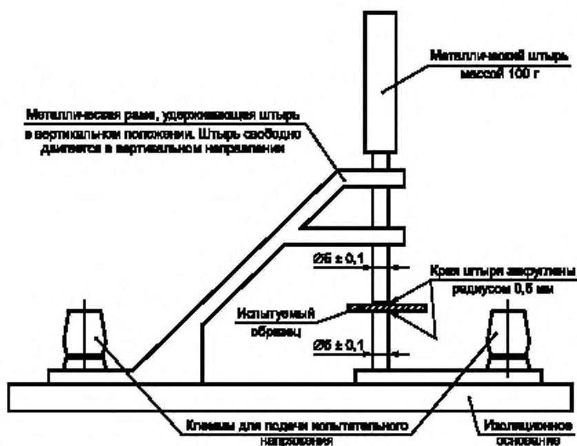
Рисунок 6 — Установка для испытаний на электрическую прочность
