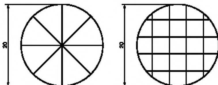
Рисунок 12 — Образец царпин для испытаний на взрывоопасность
