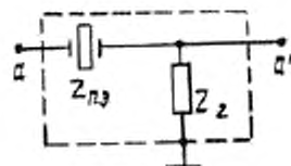
Z_{ПЭП} – проверяемый ПЭП; Z_2 – электрическая нагрузка
