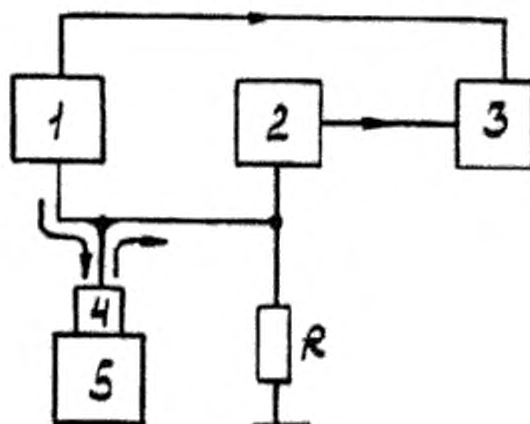
1 – генератор видеопульсов; 2 – широкополосный усилитель; 3 – осциллограф; 4 – проверяемый ПЭП; 5 – акустическая нагрузка, R – резистор сопротивлением (50 \pm 1) Ом
