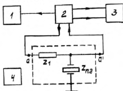
1 – частотомер; 2 – измеритель АЧХ; 3 – графопроектор; Z_{ПЭП} – проверяемый ПЭП; Z_1 – электрическая нагрузка, 4 – акустическая нагрузка
