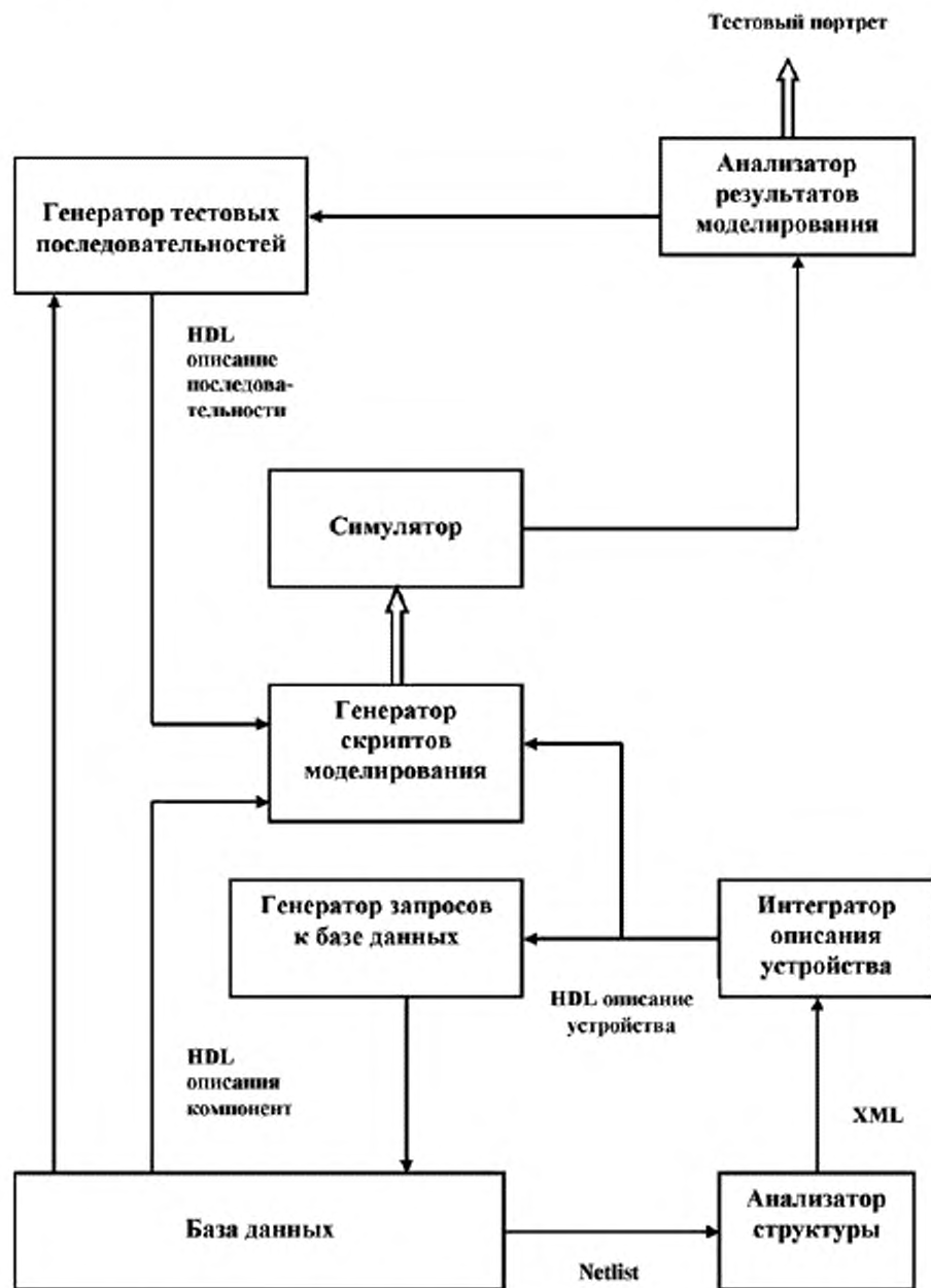
Рисунок 2 – Взаимосвязь компонентов системы автоматизированного построения тестов
