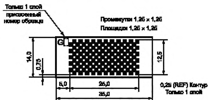
Рисунок В.11 — Тест-купон G
