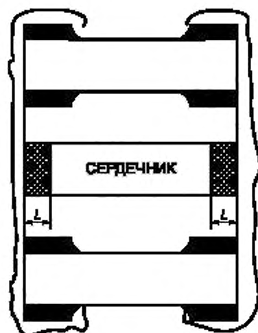
L — зазор между сердечником и металлическими поверхностями
