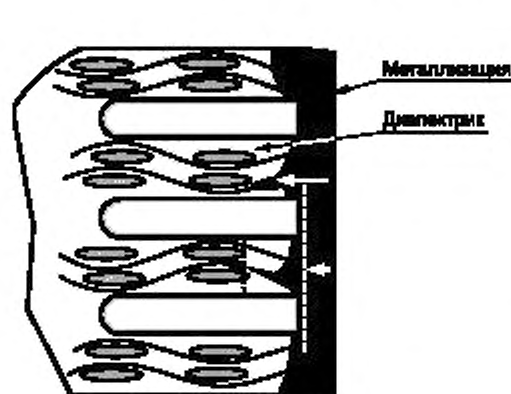
Рисунок 7 — Травление диэлектрика
