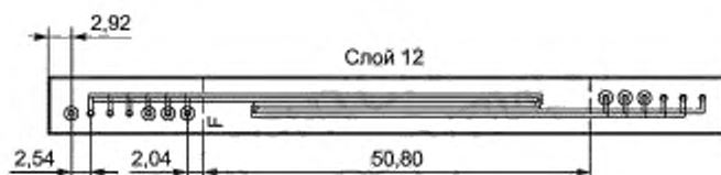
Рисунок В.15 — Тест-кулон X
