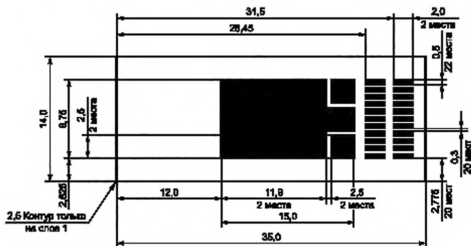
Рисунок В.12 — Тест-купон М
