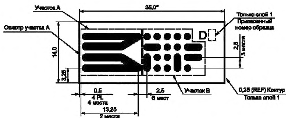
Рисунок В.4 — Тест-кулон D
