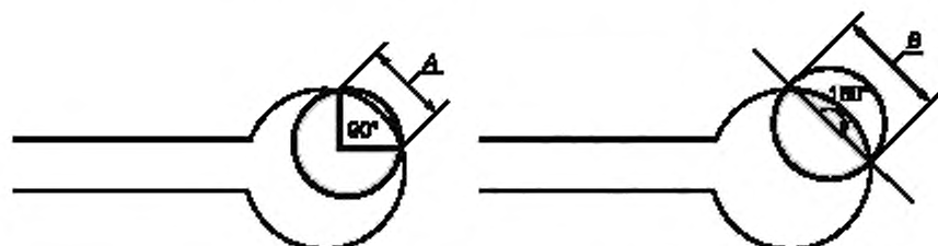
A = 1,414 · радиус сквозного металлизированного отверстия; B — диаметр сквозного металлизированного отверстия
