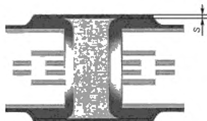
S — толщина крышки; S_1 — размер выступа крышки
