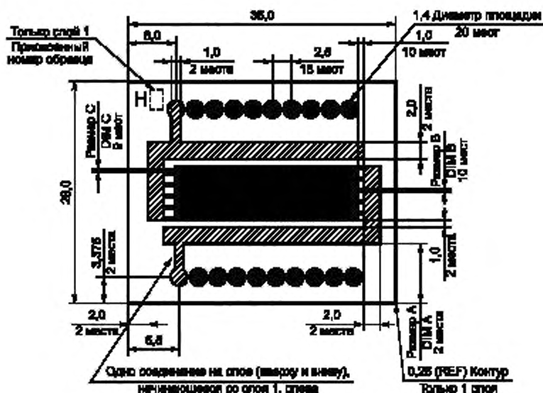
Рисунок В.7 — Тест-кулон H
