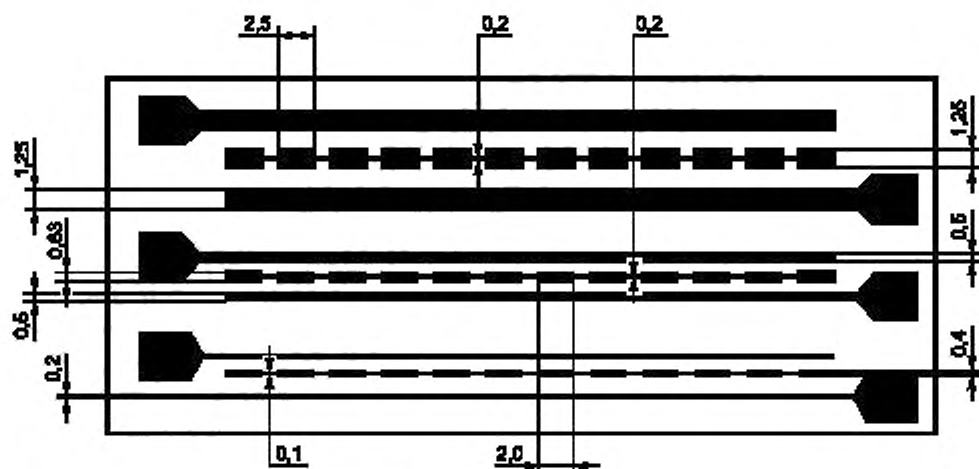
Рисунок В.13 — Тест-купон N
