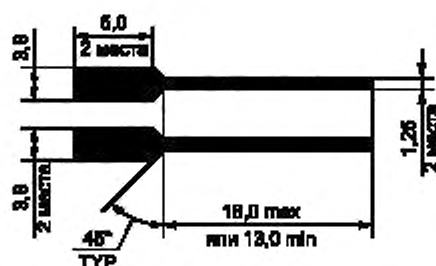
Рисунок В.3 — Тест-кулон С
