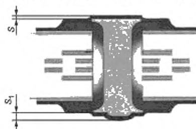
S — толщина крышки; S_1 — размер выступа крышки
