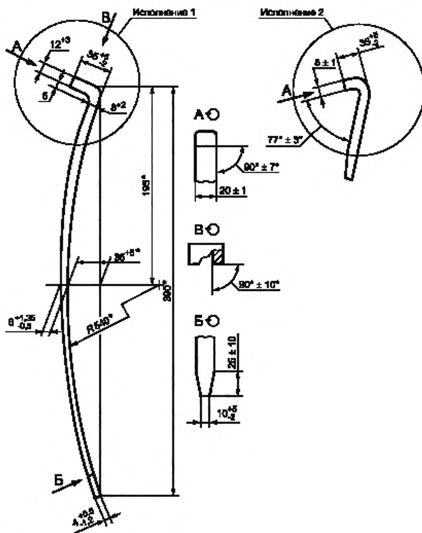
Рисунок 11 — Чека типа 1
