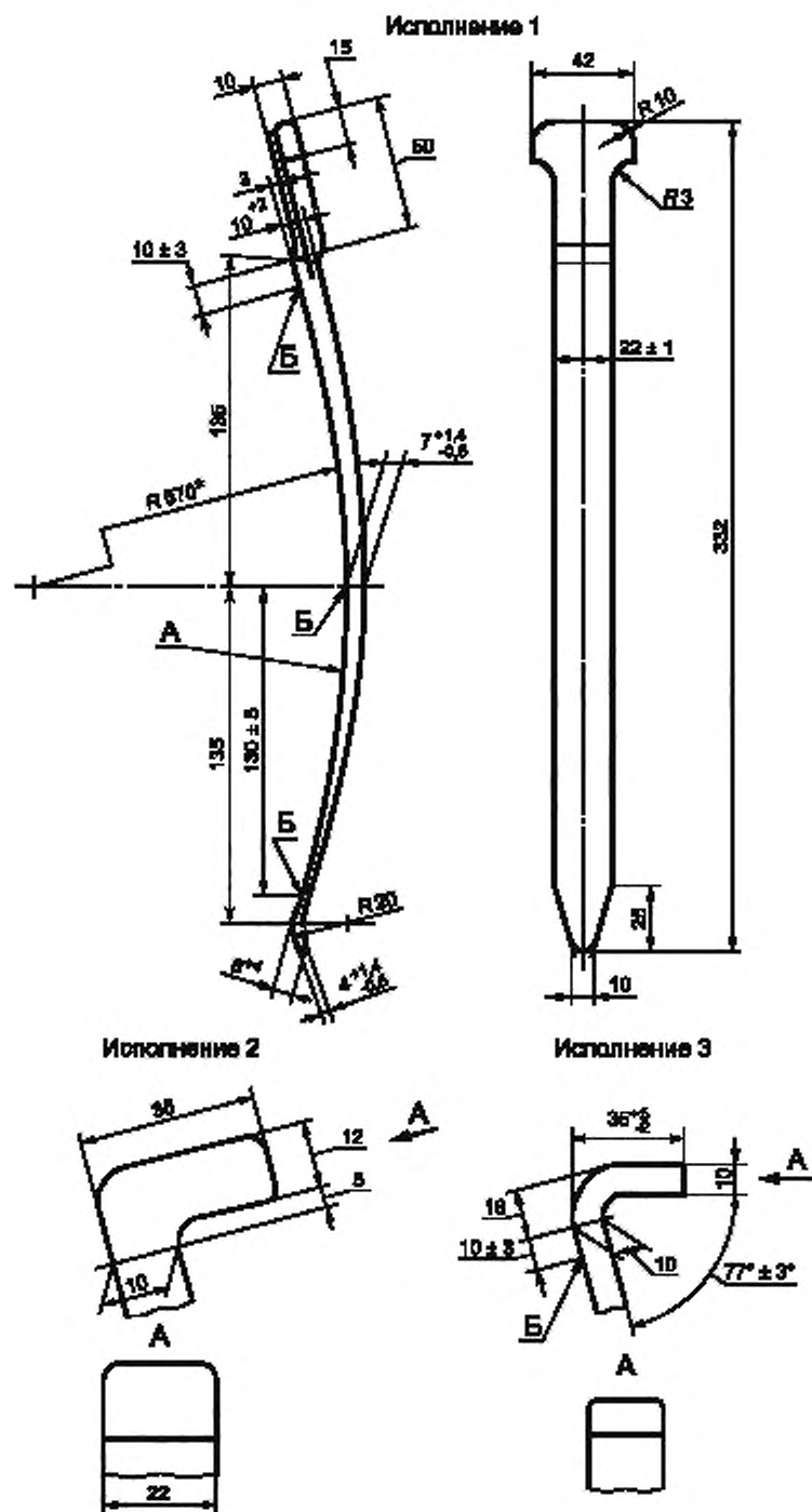
Рисунок 12 — Чека типа 2
