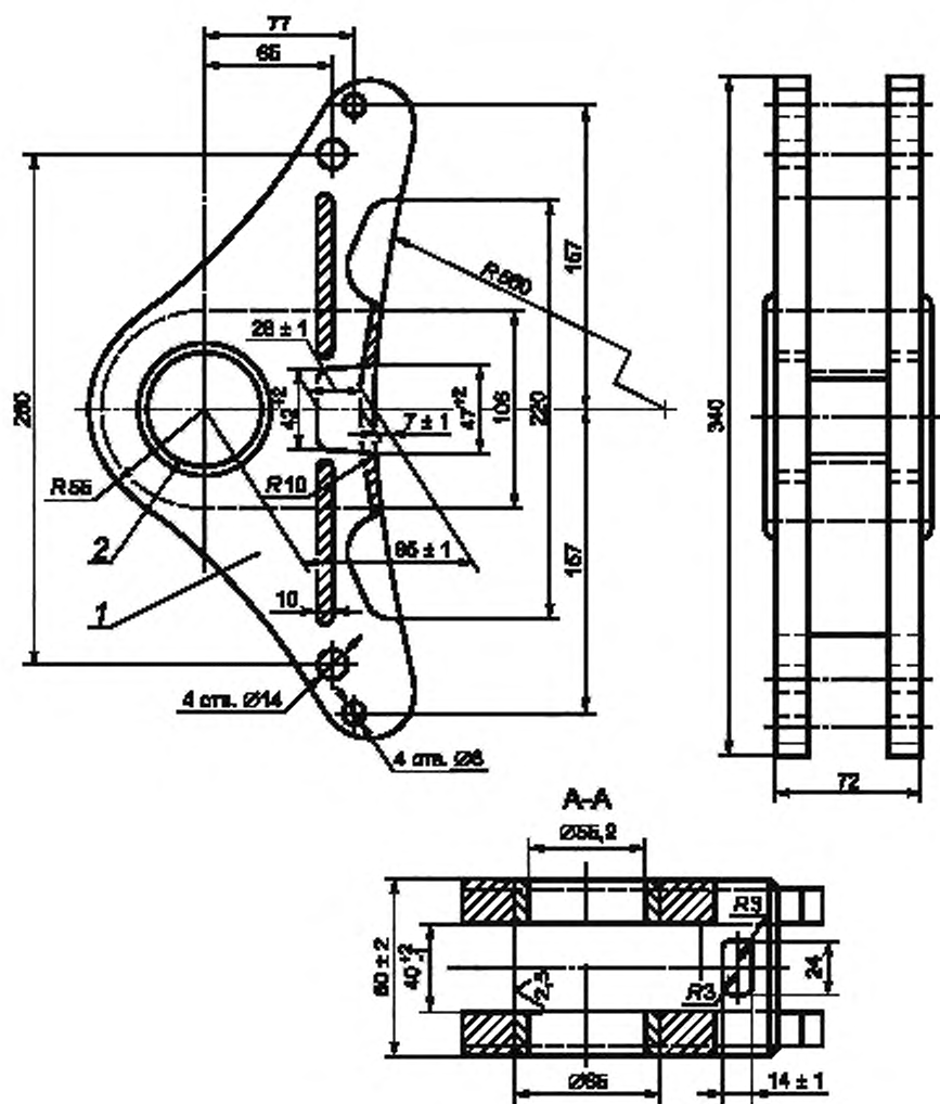
Рисунок 6 — Башмак типа 2 — Исполнение 2
