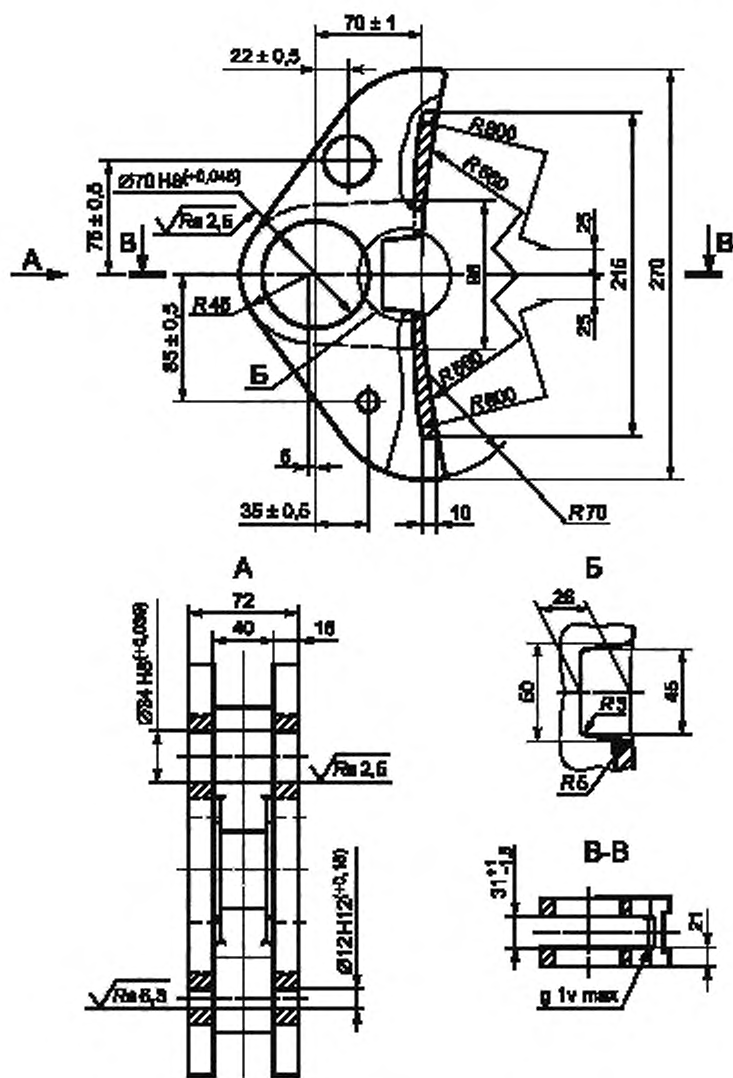
Рисунок 10 — Башмак типа 5
