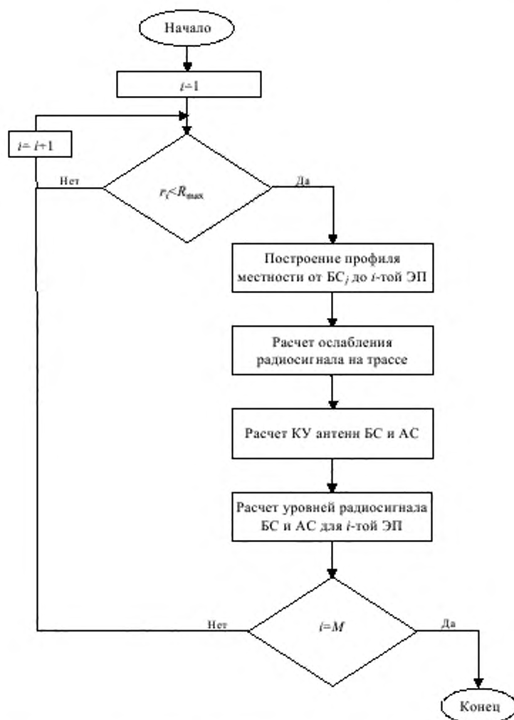
Рисунок 4.2 - Блок-схема алгоритма построения радиопокрытия БС
