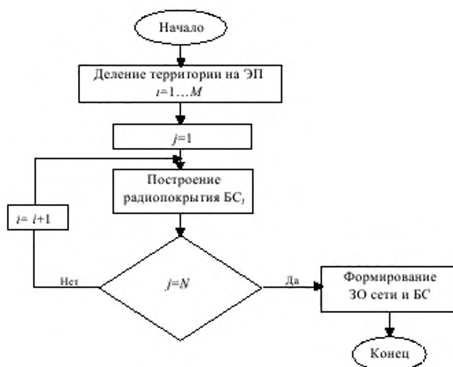
Рисунок 4.1 - Блок-схема алгоритма построения зон обслуживания
