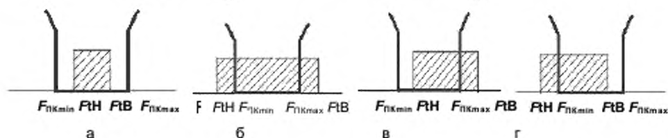
Рисунок 8.1— Положение полосы частот излучения ПРД относительно полосы пропускания побочного канала приема ПРМ
