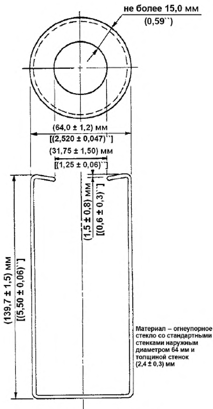
Рисунок 3 – Сосуд для образца
