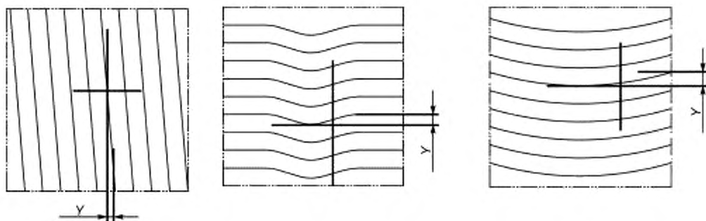
Рисунок 1 — Примеры смещения проволоки
