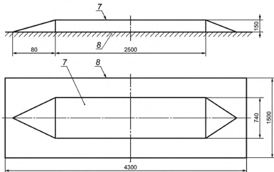
7 — перегородка; 8 — пластина заземления
