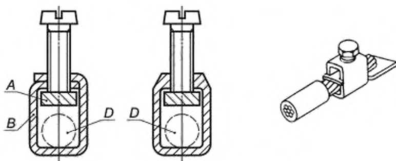
Выходы с непрямой передачей давления
