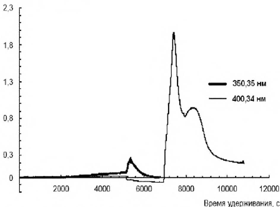
Рисунок 3 – Хроматограмма, показывающая пики удерживания фракций нафтеновых ароматических и полярных ароматических соединений
