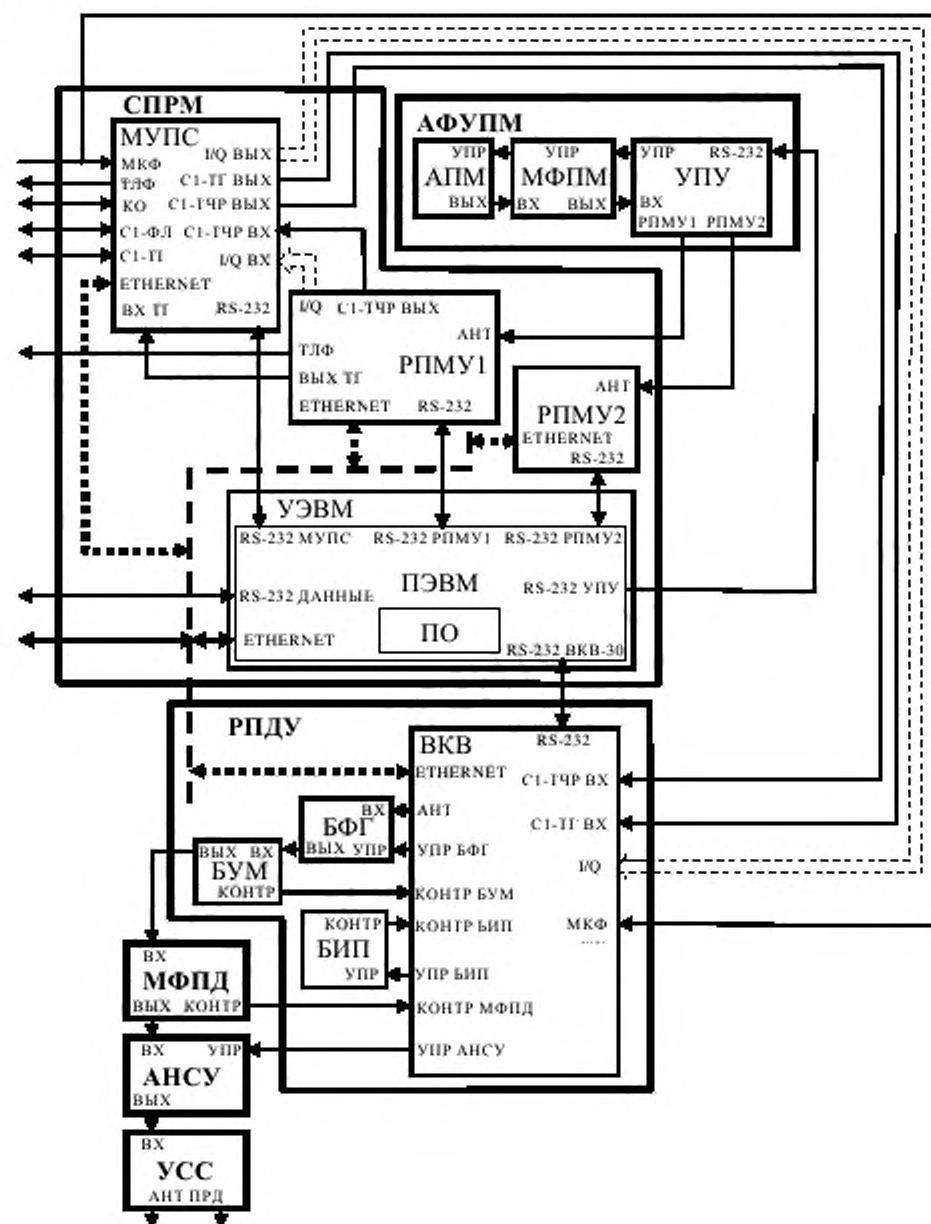
Рисунок 1 – Структура КТС ААРС
