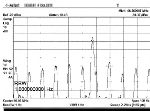
Рисунок В.39 – Полоса сканирования (Span) 100 Гц
