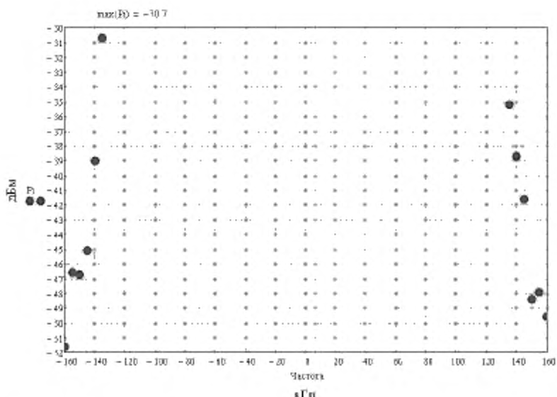
Рисунок В.34 – Разности спектральных плотностей мощности
