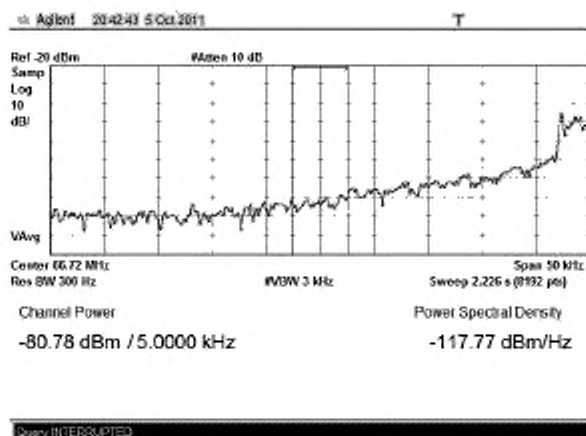
Рисунок В.24 – Плотность мощности минус 117,8 дБм/Гц на частоте f_{(0.145)}
