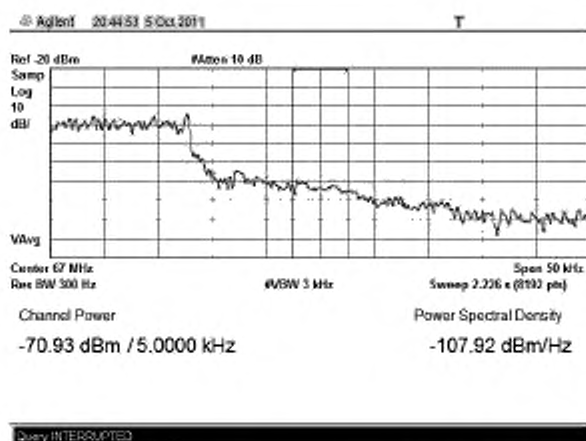
Рисунок В.28 – Плотность мощности минус 107,9 дБм/Гц на частоте f_{(0+135)}
