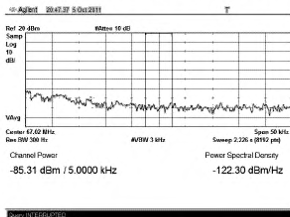
Рисунок В.33 – Плотность мощности минус 122,3 дБм/Гц на частоте f_{(0+160)}
