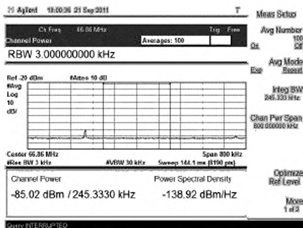
Рисунок В.15 – Измерение мощности шума
