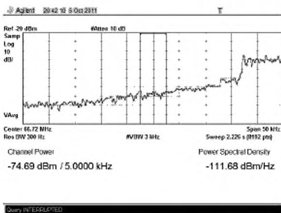
Рисунок В.25 – Плотность мощности минус 111,7 дБм/Гц на частоте f_{(0-140)}
