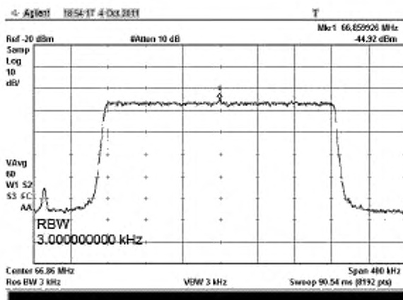
Рисунок В.35 – Полоса сканирования (Span) 400 кГц
