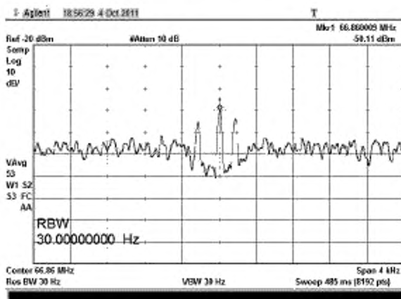
Рисунок В.37 – Полоса сканирования (Span) 4 кГц
