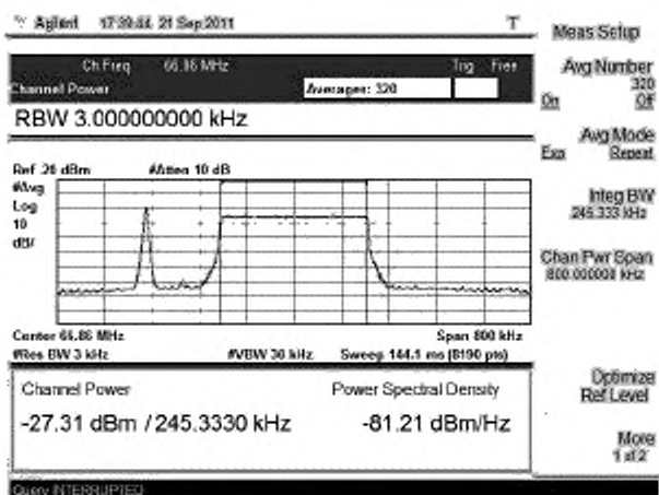
Рисунок В.11 – Сигнал для измерения мощности
