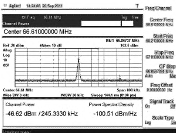
Рисунок В.13 – Измерение мощности синусоидального сигнала
