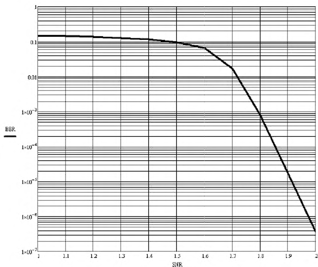
Рисунок Б.1 – График зависимости BER от ОСШ
