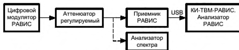
Рисунок 4 – Схема измерения чувствительности и динамического диапазона
