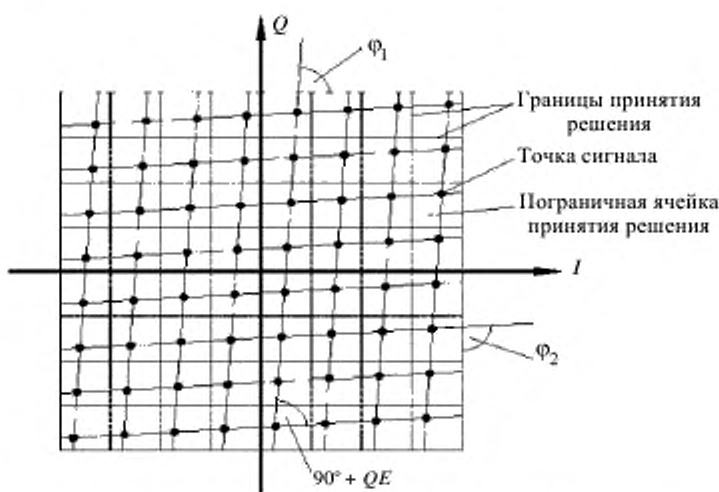
Рисунок 8 – Искажение диаграммы созвездия, вызванное квадратурной ошибкой
