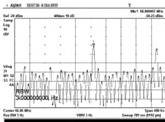
Рисунок В.38 – Полоса сканирования (Span) 400 Гц
