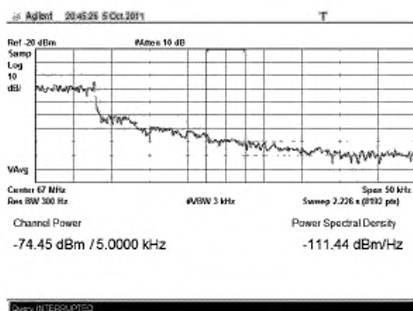
Рисунок В.29 – Плотность мощности минус 111,4 дБм/Гц на частоте f_{(0+140)}
