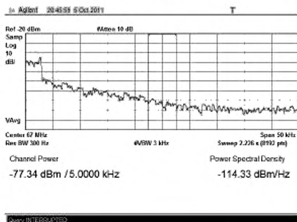
Рисунок В.30 – Плотность мощности минус 114,3 дБм/Гц на частоте f_{(0+145)}
