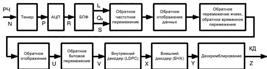
Рисунок 2 – Функциональная схема приемной части системы РАВИС (приемник)
