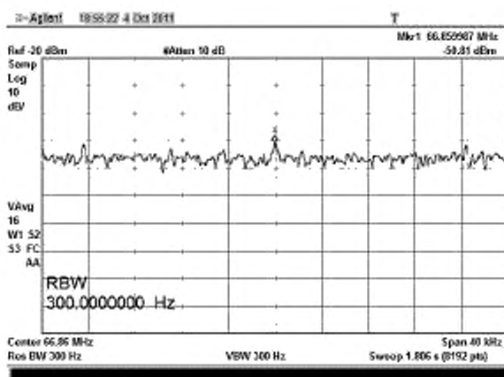
Рисунок В.36 – Полоса сканирования (Span) 40 кГц
