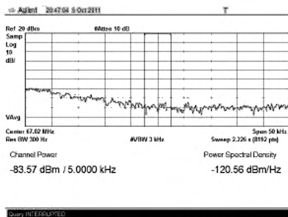
Рисунок В.32 – Плотность мощности минус 120,6 дБм/Гц на частоте f_{(0+155)}
