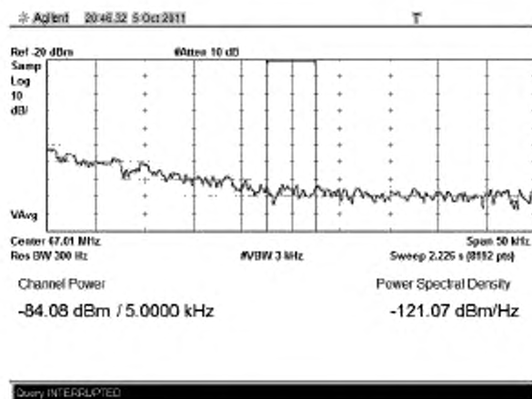
Рисунок В.31 – Плотность мощности минус 121,1 дБм/Гц на частоте f_{(0+150)}
