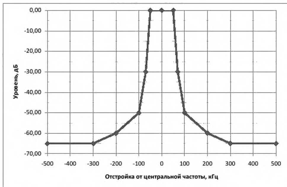
Рисунок А.1 – Маска огибающей внеполосных радиоколечаний для условной ширины полосы частот 100 кГц
