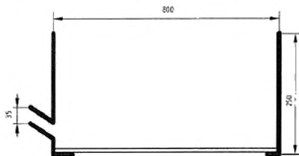
Рисунок 1 – Конструкция контейнера
